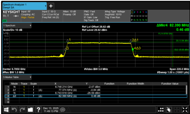
Figure 317 - 802.11ax HE80 SU LPI Minimum 99% OBW
