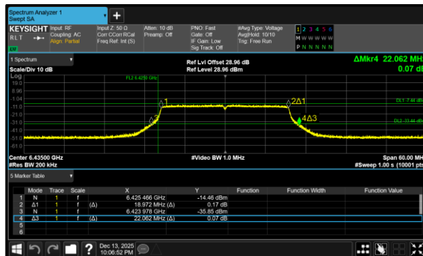
Figure 313 - 802.11ax HE20 SU LPI Minimum 99% OBW
