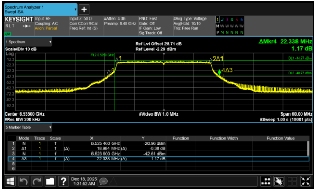
Figure 281 - 802.11ax HE20 SU VLP Minimum 99% OBW
