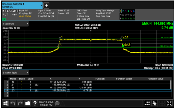
Figure 256 - 802.11ax HE160 SU LPI Maximum 99% OBW
