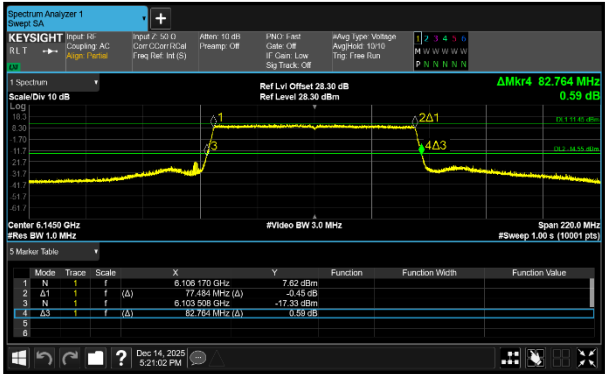
Figure 270 - 802.11ax HE80 SU SP Maximum 99% OBW
