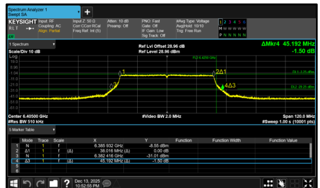
Figure 316 - 802.11ax HE40 SU LPI Maximum 99% OBW
