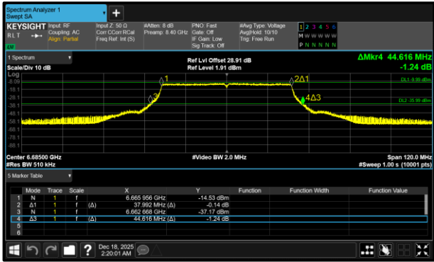
Figure 283 - 802.11ax HE40 SU VLP Minimum 99% OBW
