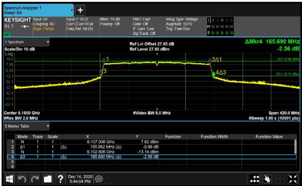
Figure 272 - 802.11ax HE160 SU SP Maximum 99% OBW
