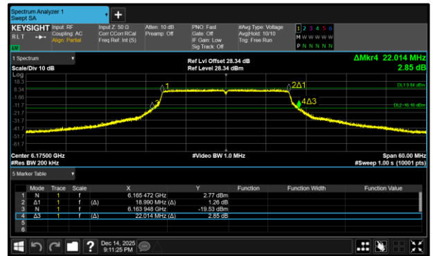
Figure 322 - 802.11ax HE20 SU SP Maximum 99% OBW
