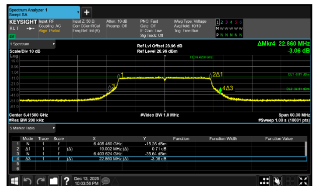
Figure 290 - 802.11ax HE20 SU LPI Maximum 26 dB EBW
