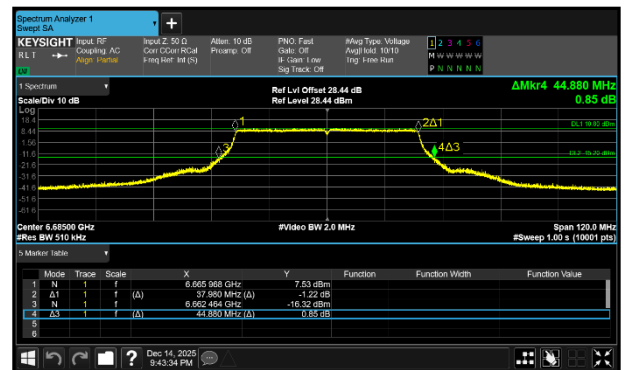
Figure 300 - 802.11ax HE40 SU SP Maximum 26 dB EBW
