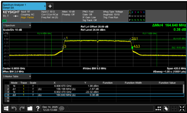
Figure 319 - 802.11ax HE160 SU LPI Minimum 99% OBW
