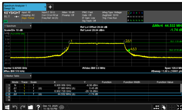
Figure 315 - 802.11ax HE40 SU LPI Minimum 99% OBW
