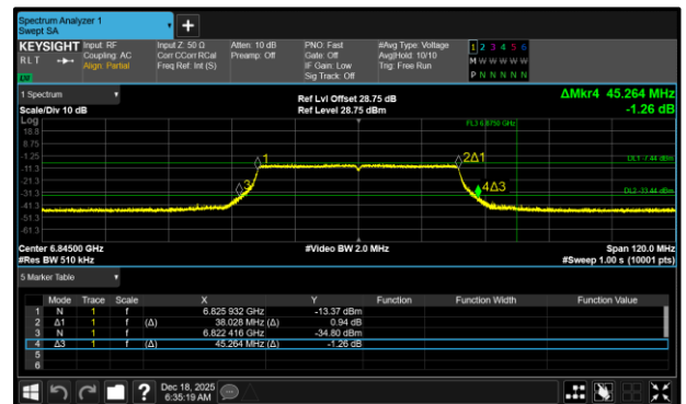
Figure 308 - 802.11ax HE40 SU VLP Maximum 26 dB EBW
