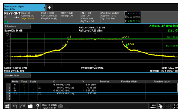
Figure 172 - 802.11ax HE40 SU SP Maximum 99% OBW
