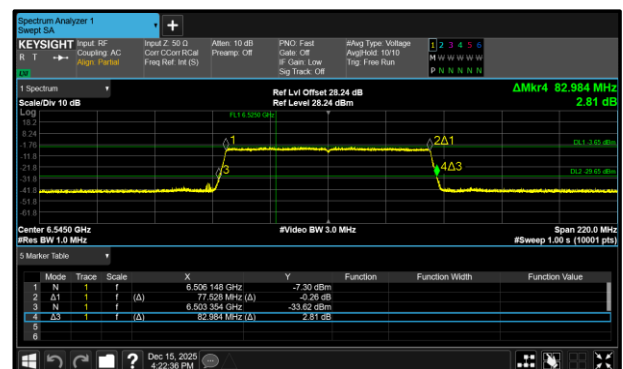
Figure 206 - 802.11ax HE80 SU LPI Maximum 26 dB EBW
