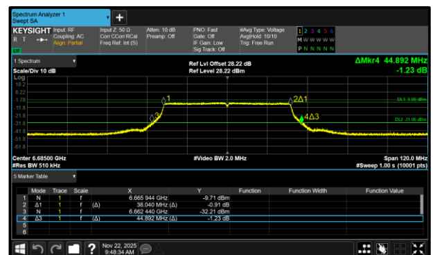
Figure 92 - 802.11ax HE40 SU VLP Maximum 99% OBW
