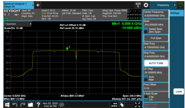
Plot 7-60 PSD Antenna WF7a (160MHz BW 802.11be(SU) - Ch.175)
