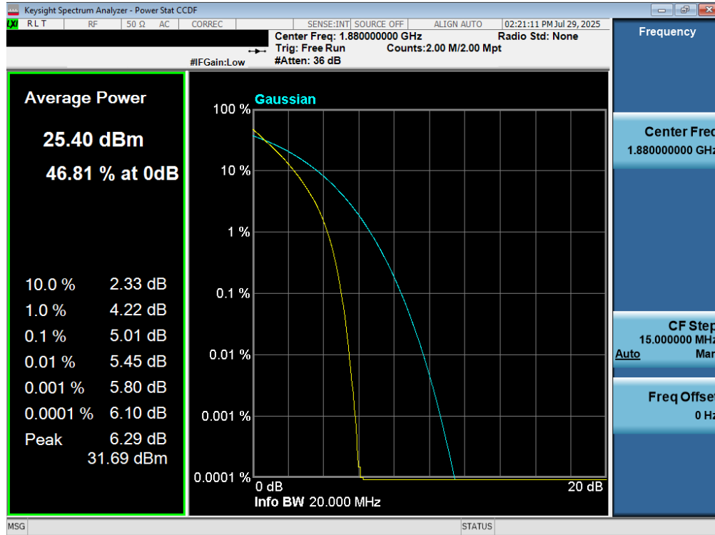
Plot 7-253. PAR Plot (LTE Band 2 - 20MHz QPSK - Full RB Configuration)
