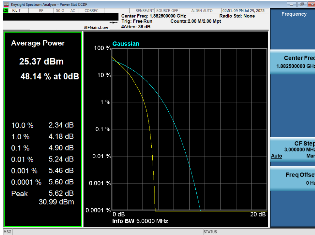
Plot 7-217. PAR Plot (LTE Band 25 - 5MHz QPSK - Full RB Configuration)
