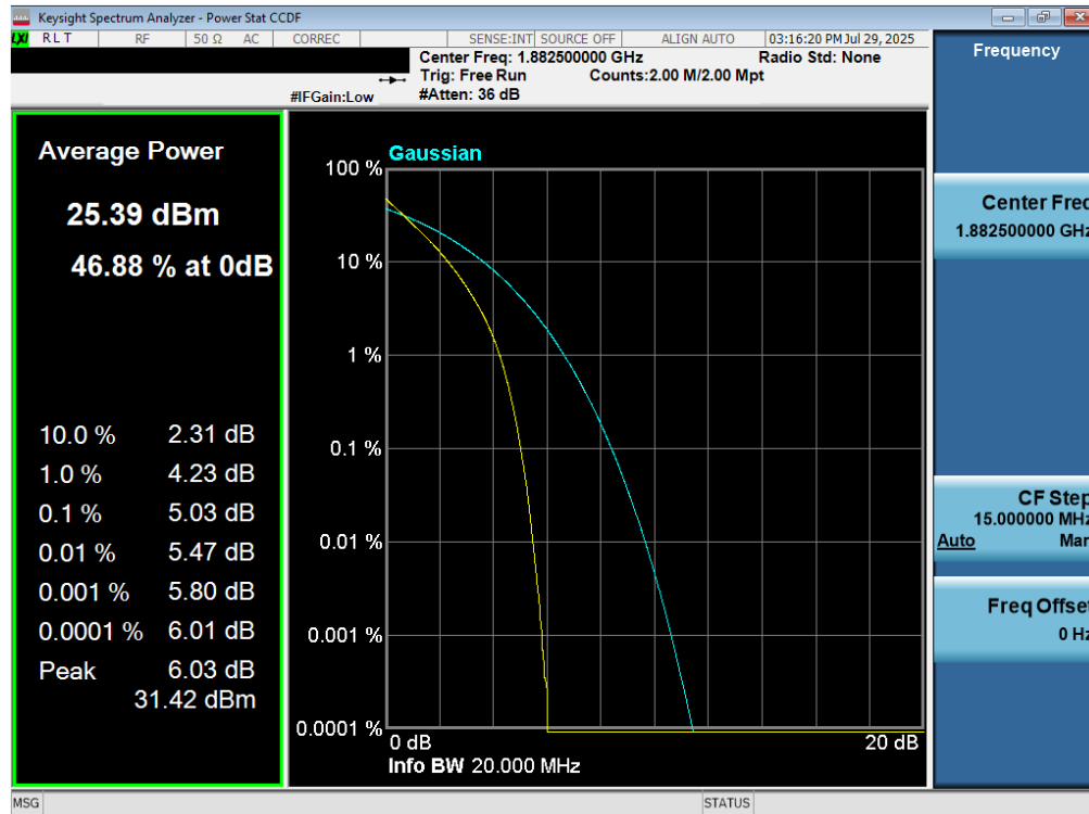
Plot 7-229. PAR Plot (LTE Band 25 - 20MHz QPSK - Full RB Configuration)
