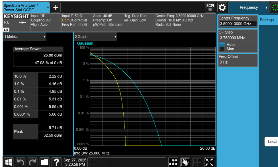
Plot 7-299. PAR Plot (NR Band n77 DoD-Band - 25MHz DFT-s-OFDM QPSK - Full RB)
