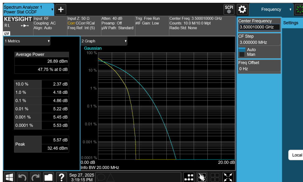
Plot 7-294. PAR Plot (NR Band n77 DoD-Band - 20MHz DFT-s-OFDM QPSK - Full RB)
