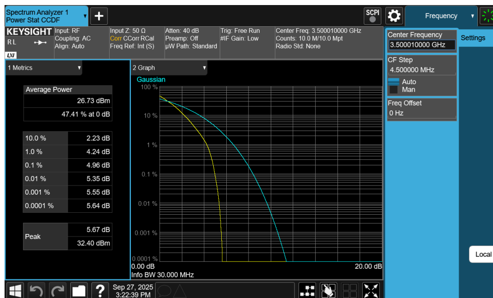
Plot 7-304. PAR Plot (NR Band n77 DoD-Band - 30MHz DFT-s-OFDM QPSK - Full RB)
