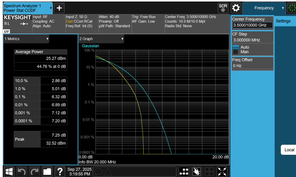
Plot 7-296. PAR Plot (NR Band n77 DoD-Band - 20MHz DFT-s-OFDM 64-QAM - Full RB)
