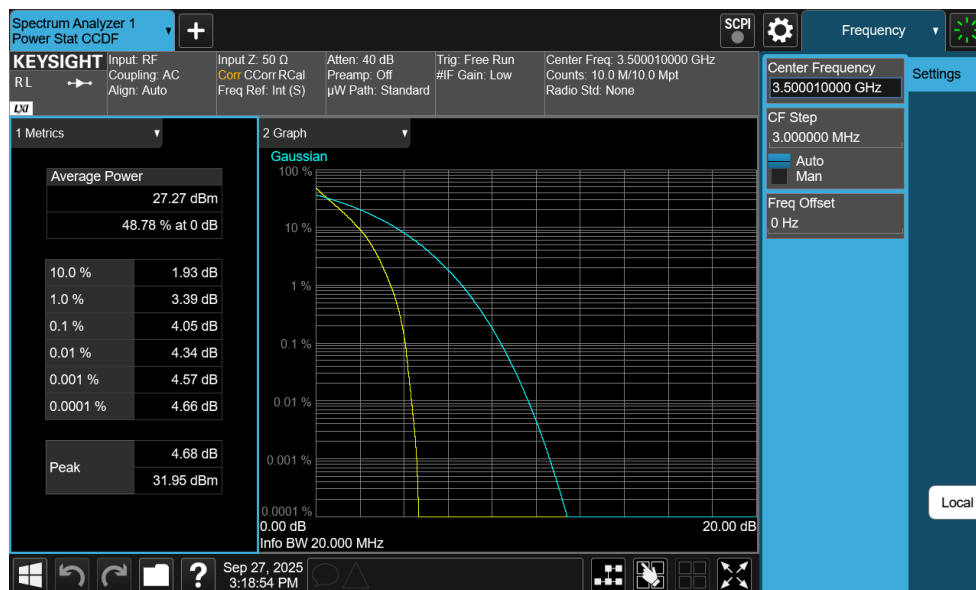
Plot 7-293. PAR Plot (NR Band n77 DoD-Band - 20MHz DFT-s-OFDM \pi/2 BPSK - Full RB)
