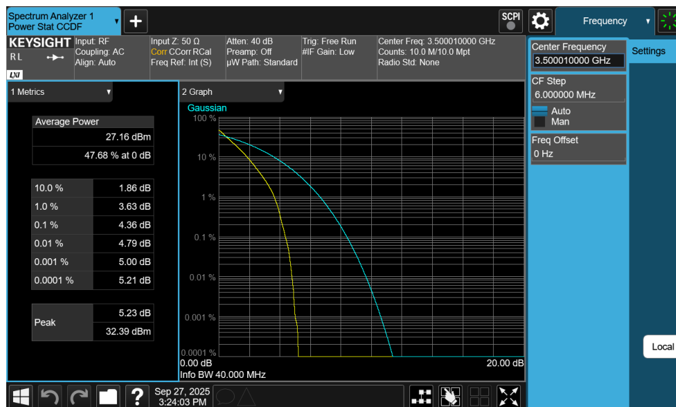
Plot 7-308. PAR Plot (NR Band n77 DoD-Band - 40MHz DFT-s-OFDM \pi/2 BPSK - Full RB)
