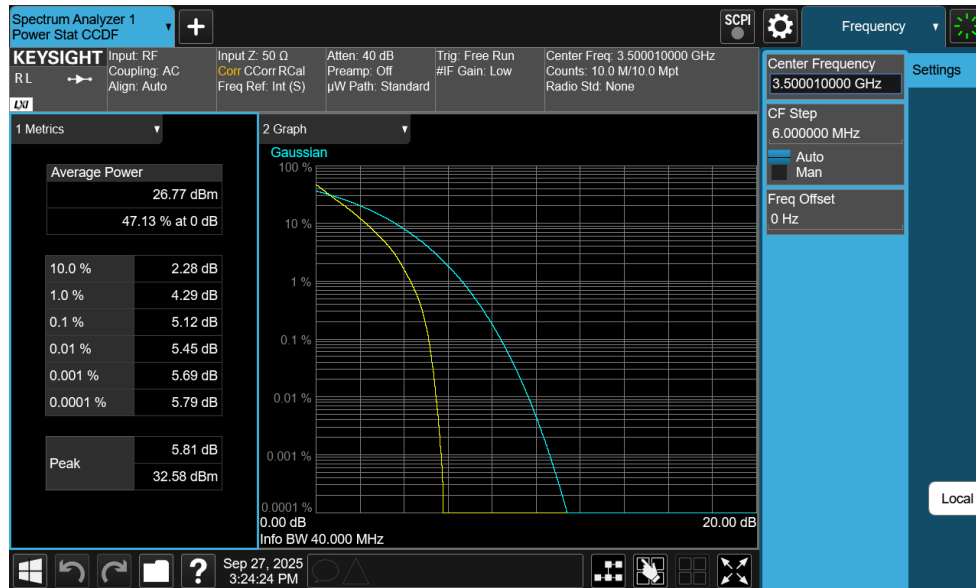
Plot 7-309. PAR Plot (NR Band n77 DoD-Band - 40MHz DFT-s-OFDM QPSK - Full RB)
