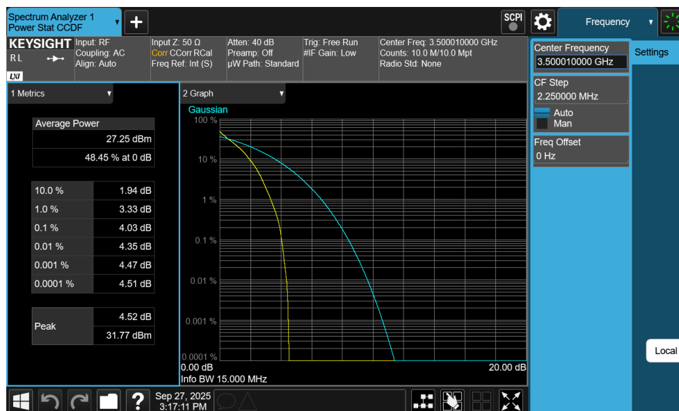
Plot 7-288. PAR Plot (NR Band n77 DoD-Band - 15MHz DFT-s-OFDM \pi/2 BPSK - Full RB)
