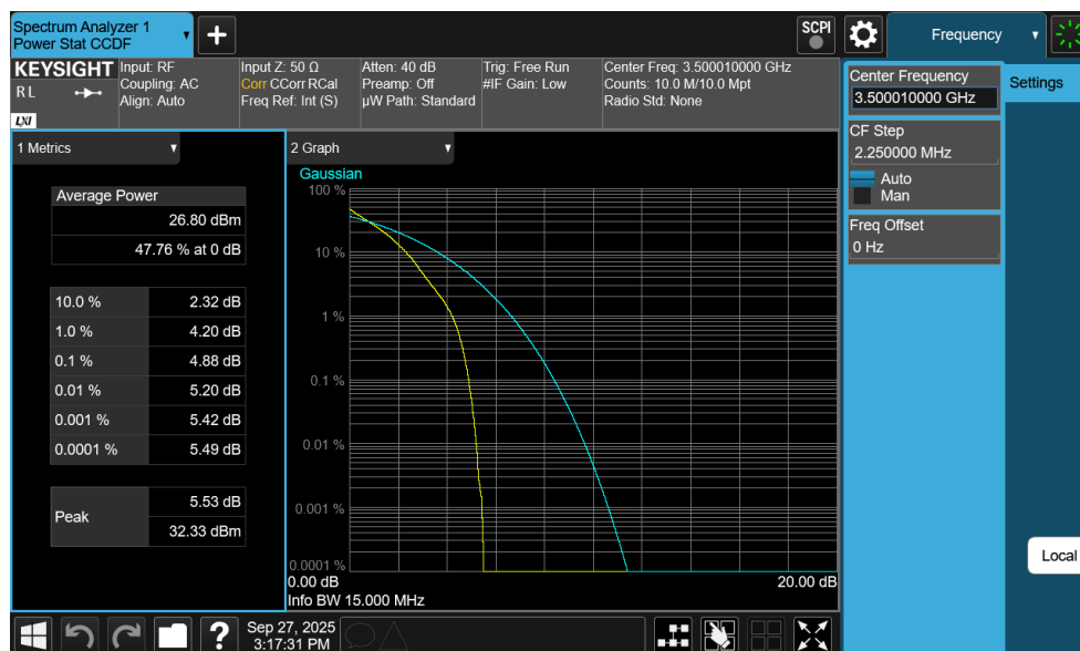
Plot 7-289. PAR Plot (NR Band n77 DoD-Band - 15MHz DFT-s-OFDM QPSK - Full RB)
