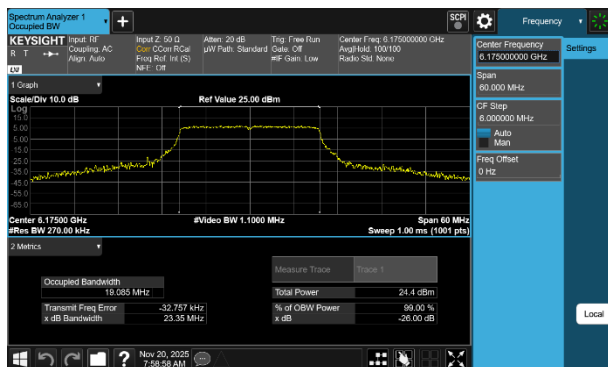
Plot 7-29 26dB BW & 99% OBW Antenna 3a (20MHz BW 802.11be(SU) - Ch.45)
