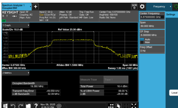
Plot 7-77 26dB BW & 99% OBW Antenna 1b (20MHz BW 802.11be(SU) - Ch.185)
