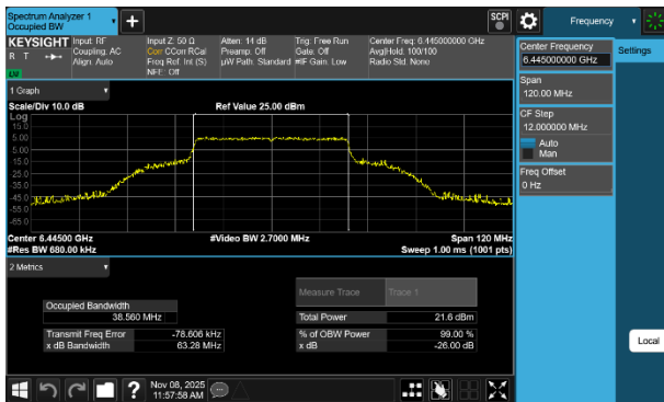
Plot 7-46 26dB BW & 99% OBW Antenna 3a (40MHz BW 802.11be(SU) - Ch.99)
