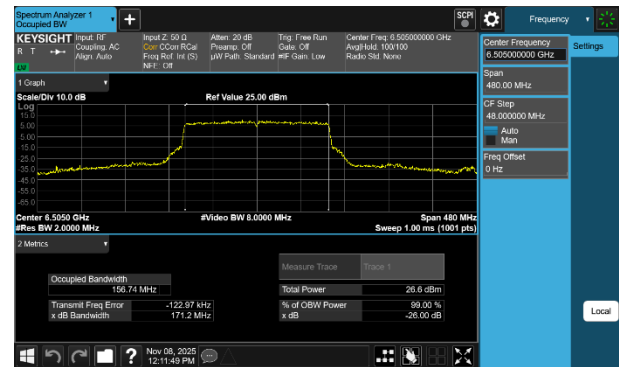
Plot 7-48 26dB BW & 99% OBW Antenna 3a (160MHz BW 802.11be(SU) - Ch.111)
