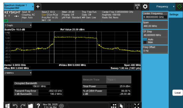
Plot 7-84 26dB BW & 99% OBW Antenna 1b (160MHz BW 802.11be(SU) - Ch.207)
