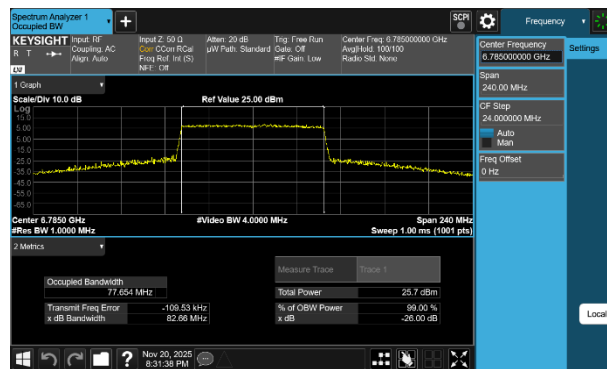
Plot 7-67 26dB BW & 99% OBW Antenna 1b (80MHz BW 802.11be(SU) - Ch.167)
