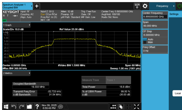
Plot 7-81 26dB BW & 99% OBW Antenna 1b (20MHz BW 802.11be(SU) - Ch.189)
