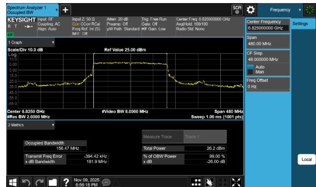
Plot 7-80 26dB BW & 99% OBW Antenna 1b (160MHz BW 802.11be(SU) - Ch.175)
