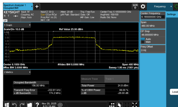
Plot 7-32 26dB BW & 99% OBW Antenna 3a (160MHz BW 802.11be(SU) - Ch.47)
