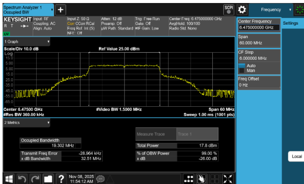
Plot 7-45 26dB BW & 99% OBW Antenna 3a (20MHz BW 802.11be(SU) - Ch.105)
