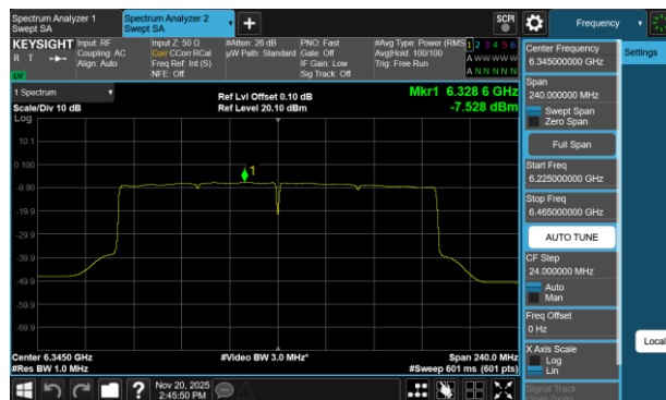
Plot 7-68 PSD Antenna 3a (160MHz BW 802.11be(SU) - Ch.79)
