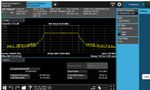
Plot 7-30 26dB BW & 99% OBW Antenna 3a (40MHz BW 802.11be(SU) - Ch.187)
