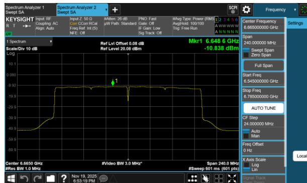
Plot 7-60 PSD Antenna 3c (160MHz BW 802.11be(SU) - Ch.143)
