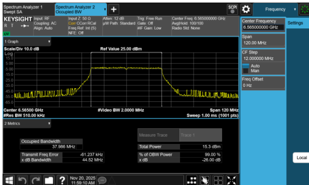
Plot 7-26 26dB BW & 99% OBW Antenna 3a (40MHz BW 802.11be(SU) - Ch.123)
