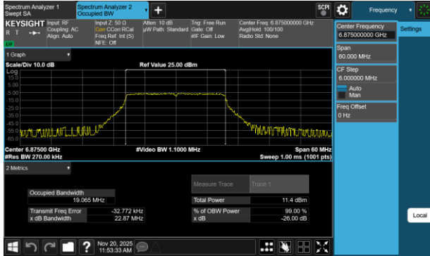
Plot 7-25 26dB BW & 99% OBW Antenna 3a (20MHz BW 802.11be(SU) - Ch.185)
