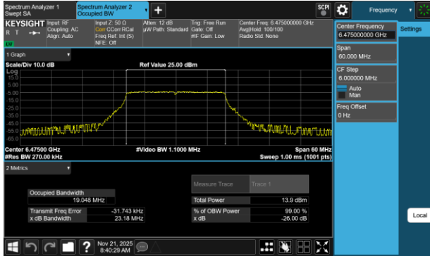
Plot 7-37 26dB BW & 99% OBW Antenna 1b (20MHz BW 802.11be(SU) - Ch.105)
