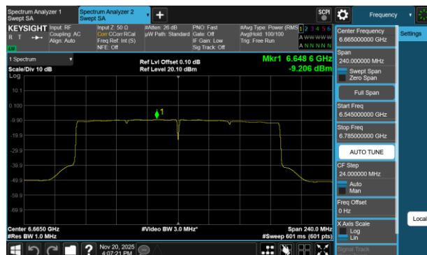
Plot 7-76 PSD Antenna 3a (160MHz BW 802.11be(SU) - Ch.143)
