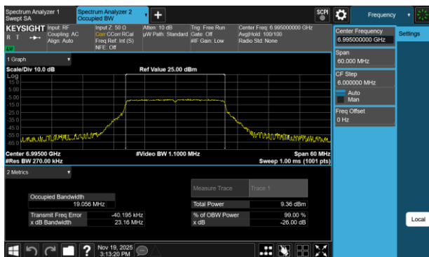
Plot 7-13 26dB BW & 99% OBW Antenna 3c (20MHz BW 802.11be(SU) - Ch.209)
