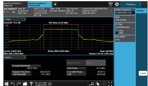
Plot 7-32 26dB BW & 99% OBW Antenna 3a (160MHz BW 802.11be(SU) - Ch.207)
