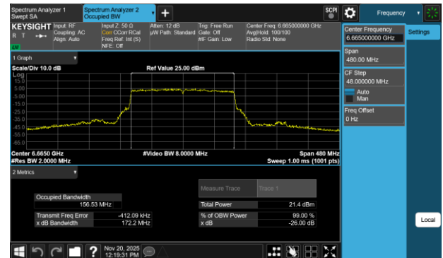
Plot 7-28 26dB BW & 99% OBW Antenna 3a (160MHz BW 802.11be(SU) - Ch.143)
