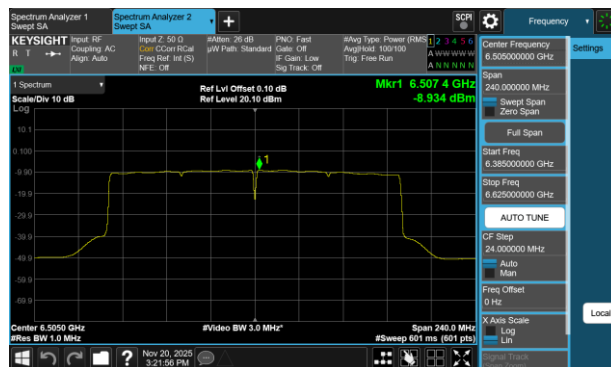
Plot 7-72 PSD Antenna 3a (160MHz BW 802.11be(SU) - Ch.111)
