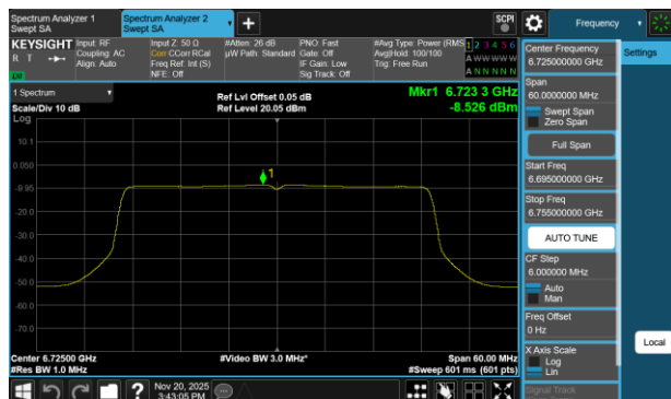
Plot 7-74 PSD Antenna 3a (40MHz BW 802.11be(SU) - Ch.155)
