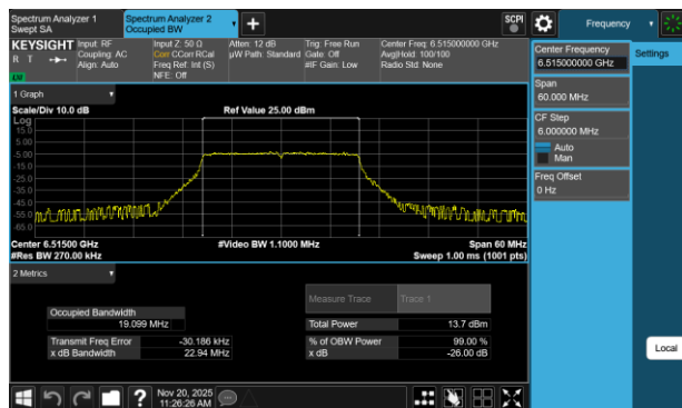
Plot 7-21 26dB BW & 99% OBW Antenna 3a (20MHz BW 802.11be(SU) - Ch.113)
