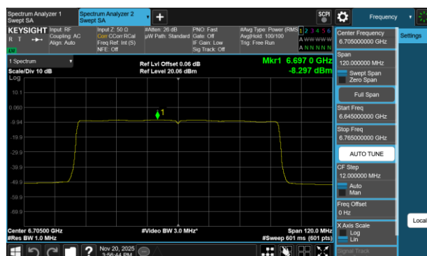
Plot 7-75 PSD Antenna 3a (80MHz BW 802.11be(SU) - Ch.151)
