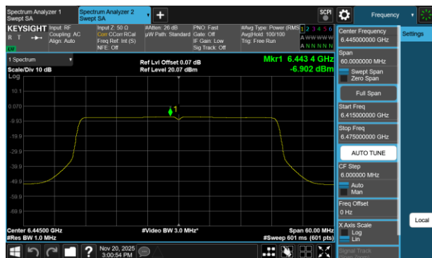
Plot 7-70 PSD Antenna 3a (40MHz BW 802.11be(SU) - Ch.99)
