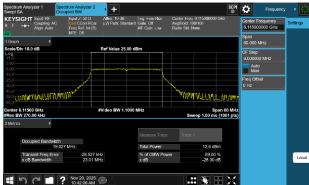
Plot 7-17 26dB BW & 99% OBW Antenna 3a (20MHz BW 802.11be(SU) - Ch.33)
