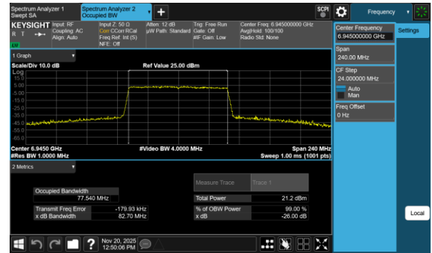
Plot 7-31 26dB BW & 99% OBW Antenna 3a (80MHz BW 802.11be(SU) - Ch.199)
