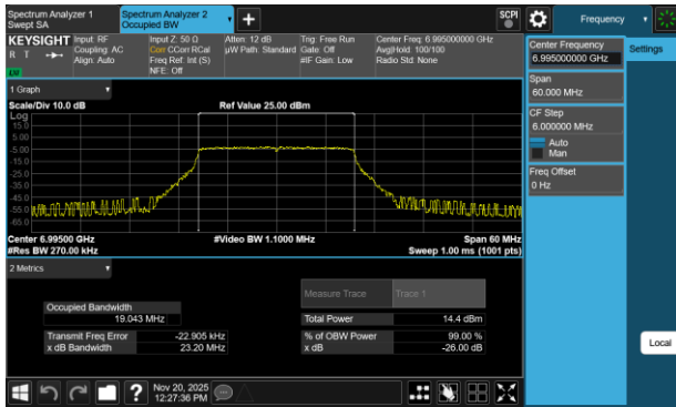
Plot 7-29 26dB BW & 99% OBW Antenna 3a (20MHz BW 802.11be(SU) - Ch.209)
