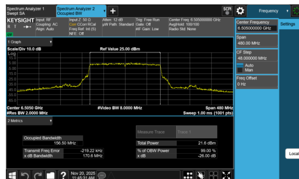
Plot 7-24 26dB BW & 99% OBW Antenna 3a (160MHz BW 802.11be(SU) - Ch.111)
