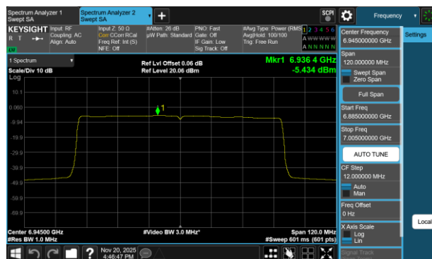
Plot 7-79 PSD Antenna 3a (80MHz BW 802.11b(SU) - Ch.199)
