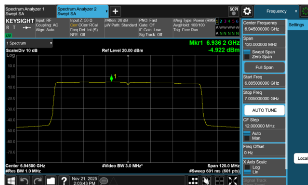
Plot 7-95 PSD Antenna 1b (80MHz BW 802.11be(SU) - Ch.199)
