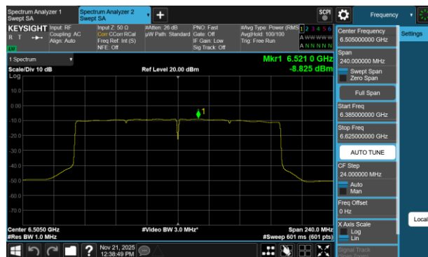
Plot 7-88 PSD Antenna 1b (160MHz BW 802.11be(SU) - Ch.111)
