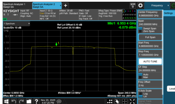
Plot 7-80 PSD Antenna 3a (160MHz BW 802.11b(SU) - Ch.207)
