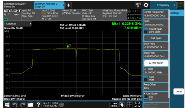
Plot 7-84 PSD Antenna 1b (160MHz BW 802.11b(SU) - Ch.79)
