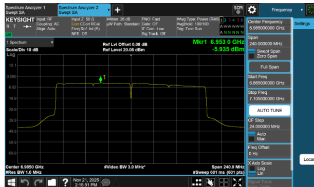
Plot 7-96 PSD Antenna 1b (160MHz BW 802.11be(SU) - Ch.207)
