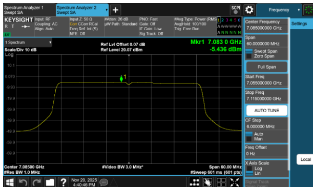
Plot 7-78 PSD Antenna 3a (40MHz BW 802.11b(SU) - Ch.227)
