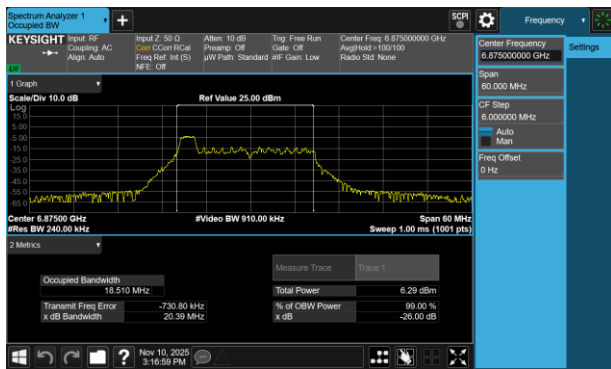
Plot 7-56 26dB BW & 99% OBW Antenna 3c (20MHz BW 802.11be(RU) RU26 Index0 - Ch.185)
