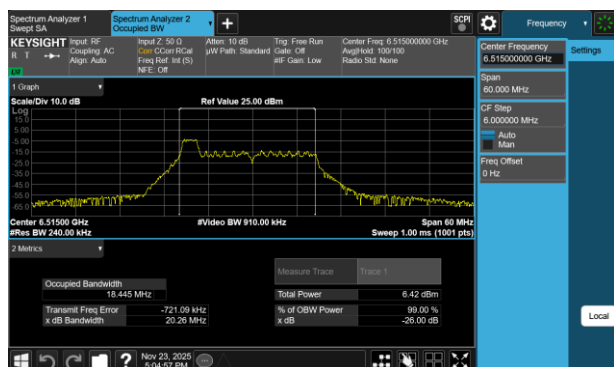
Plot 7-56 26dB BW & 99% OBW Antenna 3a (20MHz BW 802.11be(RU) RU26 Index0 - Ch.113)
