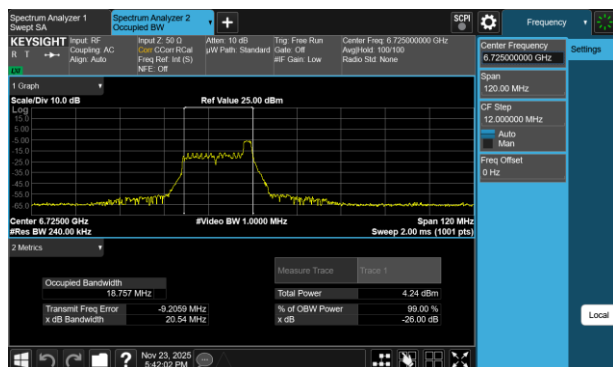
Plot 7-68 26dB BW & 99% OBW Antenna 3a (40MHz BW 802.11be(RU) RU26 Index8 - Ch.155)
