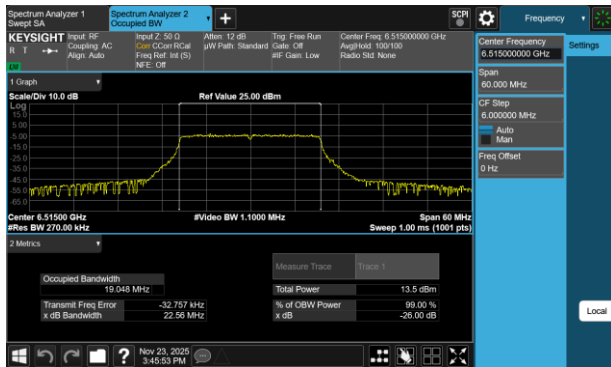
Plot 7-63 26dB BW & 99% OBW Antenna 3a (20MHz BW 802.11be(RU) RU242 Index61 - Ch.113)
