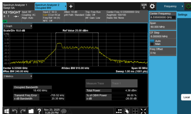
Plot 7-67 26dB BW & 99% OBW Antenna 3a (20MHz BW 802.11be(RU) RU26 Index0 - Ch.117)
