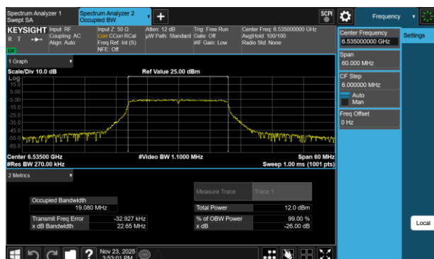
Plot 7-74 26dB BW & 99% OBW Antenna 3a (20MHz BW 802.11be(RU) RU242 Index61 - Ch.117)
