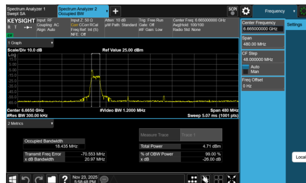
Plot 7-70 26dB BW & 99% OBW Antenna 3a (160MHz BW 802.11be(RU) RU26 Index0 - Ch.143)
