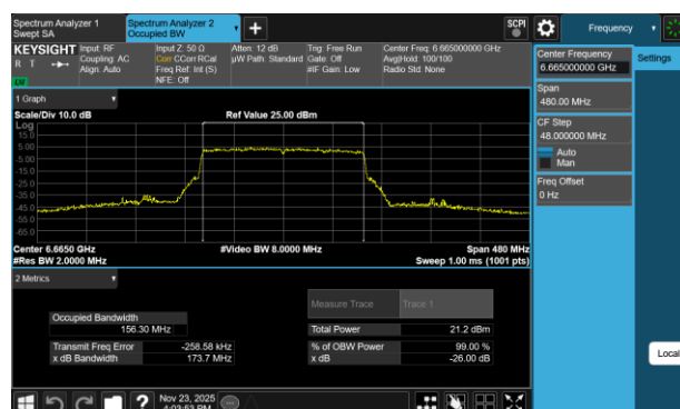
Plot 7-77 26dB BW & 99% OBW Antenna 3a (160MHz BW 802.11be(RU) RU996X2 Index68 - Ch.143)
