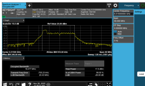
Plot 7-89 26dB BW & 99% OBW Antenna 3a (20MHz BW 802.11be(RU) RU26 Index0 - Ch.113)
