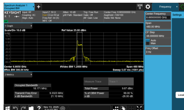
Plot 7-136 26dB BW & 99% OBW Antenna 3a (160MHz BW 802.11be(RU) RU26 Index0 - Ch.143)
