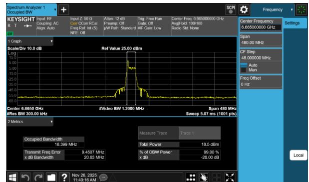
Plot 7-103 26dB BW & 99% OBW Antenna 3a (160MHz BW 802.11be(RU) RU26 Index0 - Ch.143)
