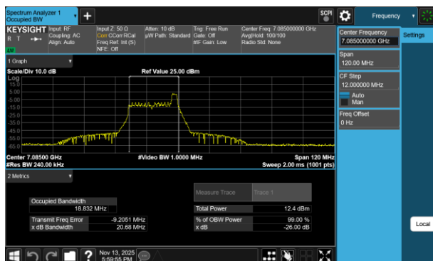
Plot 7-145 26dB BW & 99% OBW Antenna 3a (40MHz BW 802.11be(RU) RU26 Index8 - Ch.227)
