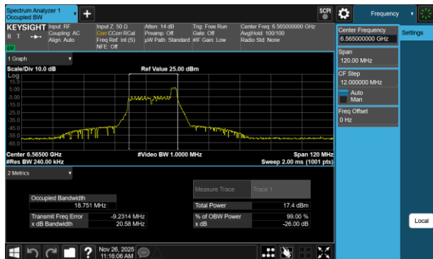
Plot 7-101 26dB BW & 99% OBW Antenna 3a (40MHz BW 802.11be(RU) RU26 Index8 - Ch.123)
