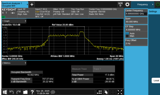
Plot 7-100 26dB BW & 99% OBW Antenna 3a (20MHz BW 802.11be(RU) RU26 Index8 - Ch.149)
