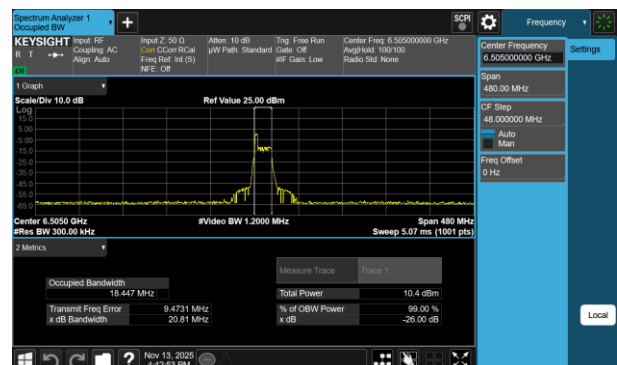
Plot 7-125 26dB BW & 99% OBW Antenna 3a (160MHz BW 802.11be(RU) RU26 Index0 - Ch.111)
