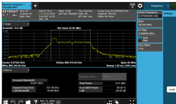
Plot 7-133 26dB BW & 99% OBW Antenna 3a (20MHz BW 802.11be(RU) RU26 Index0 - Ch.185)
