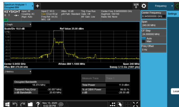
Plot 7-146 26dB BW & 99% OBW Antenna 3a (80MHz BW 802.11be(RU) RU26 Index0 - Ch.199)
