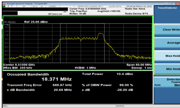
Plot 7-122 26dB BW & 99% OBW Antenna 3a (20MHz BW 802.11be(RU) RU26 Index8 - Ch.113)
