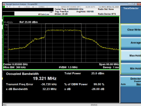
Plot 7-184 26dB BW & 99% OBW Antenna 1b (20MHz BW 802.11be(RU) RU242 Index61 - Ch.181)
