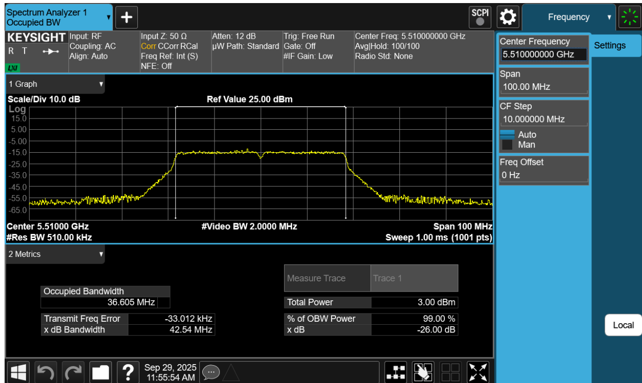
Plot 7-6 26dB BW & 99% OBW Antenna 3a (40MHz BW 802.11n - Ch.102)
