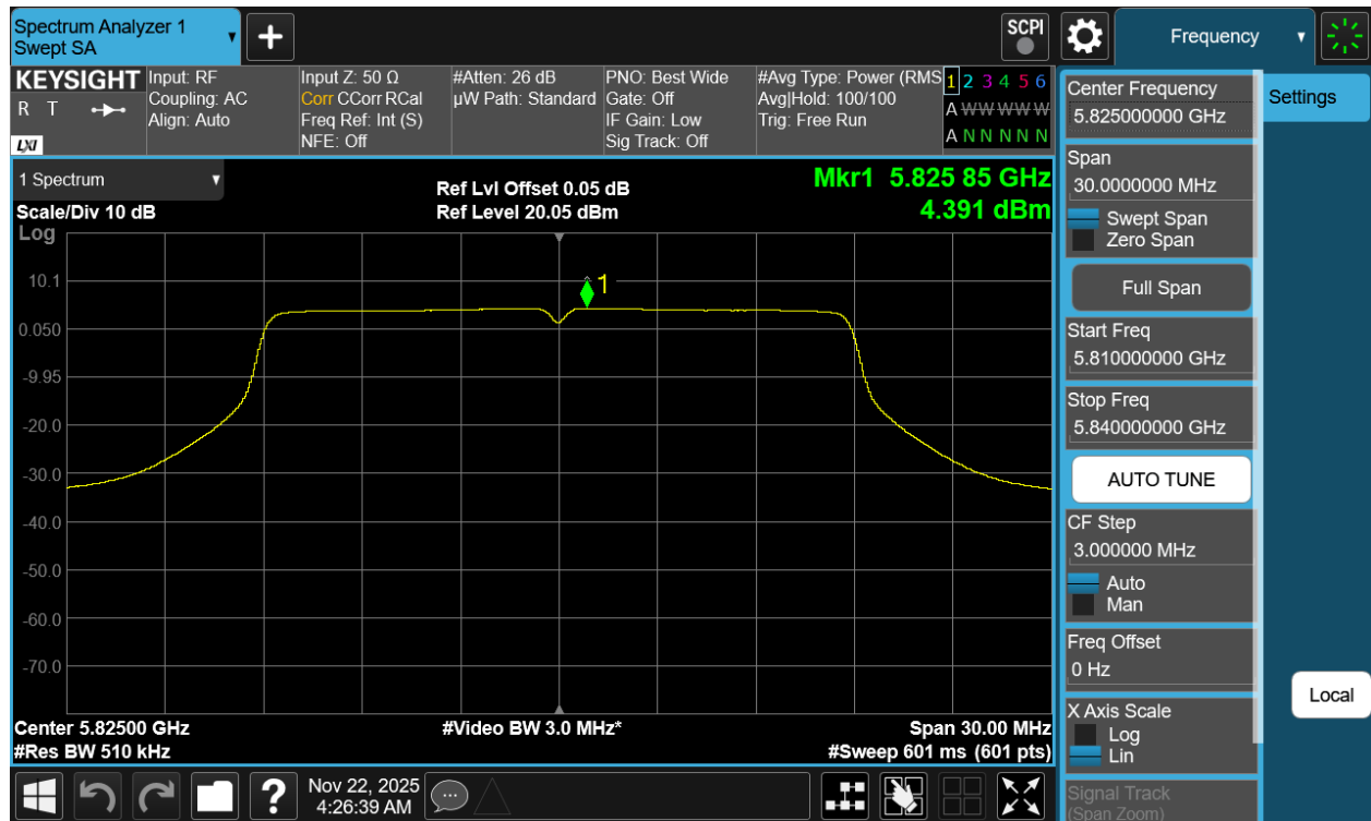
Plot 7-37 PSD Antenna 3a (20MHz BW 802.11a - Ch.165)
