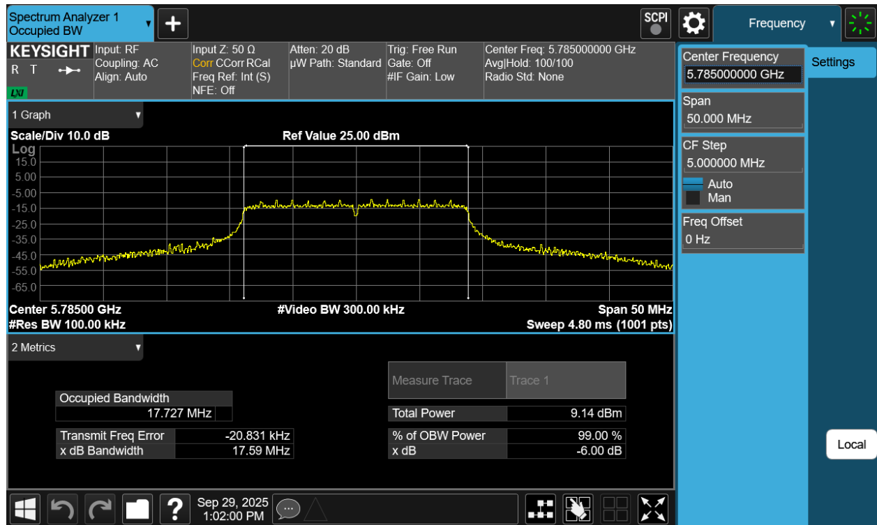
Plot 7-16 6dB OBW Antenna 3a (20MHz BW 802.11n - Ch.157)
