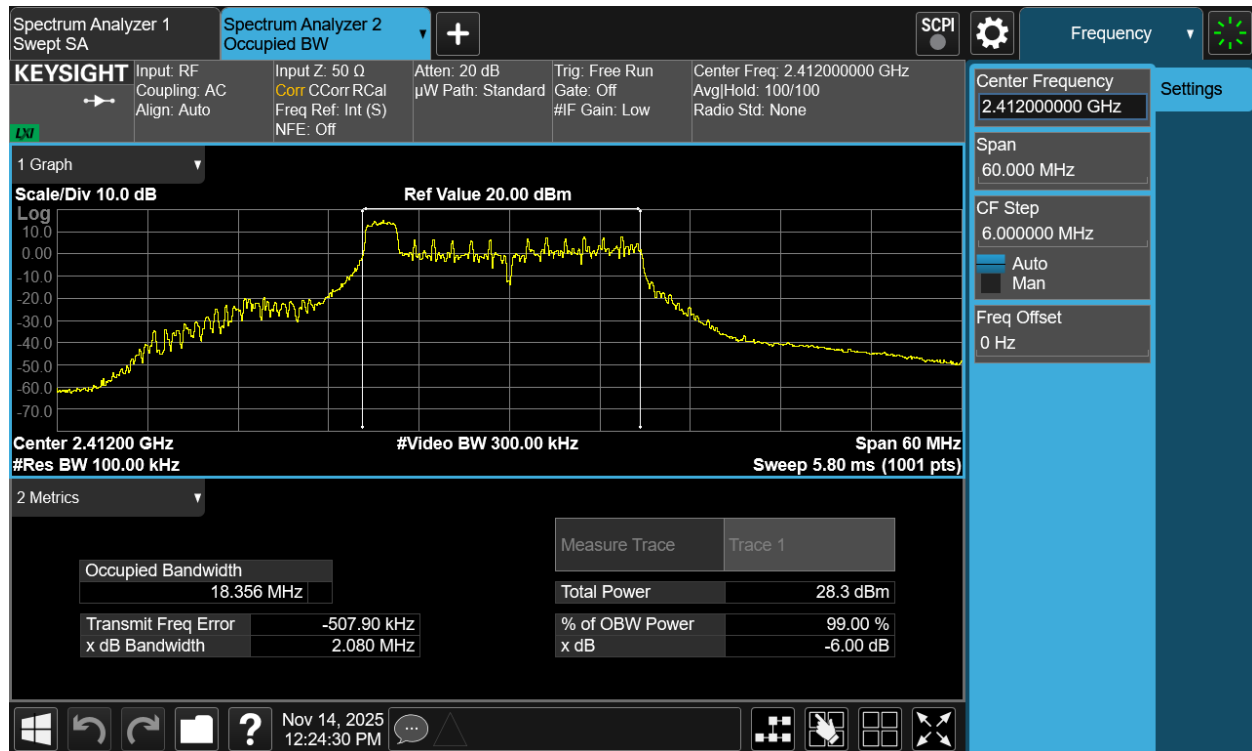
Plot 7-13 6dB BW Antenna 1a (20MHz BW 802.11be(RU) RU26 Index0 - Ch.1)
