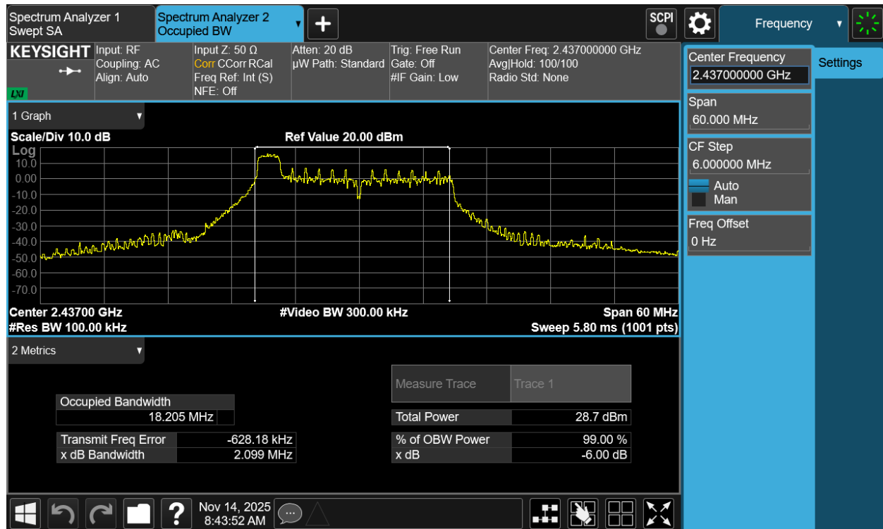
Plot 7-9 6dB BW Antenna 3a (20MHz BW 802.11be(RU) RU26 Index0 - Ch.6)
