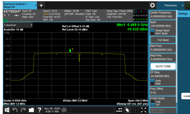
Plot 7-56 PSD Antenna WF7a (160MHz BW 802.11b(SU) - Ch.111)
