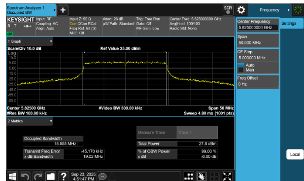
Plot 7-55 6dB OBW Antenna WF7b (20MHz BW 802.11be(RU) RU242 Index61 - Ch.165)
