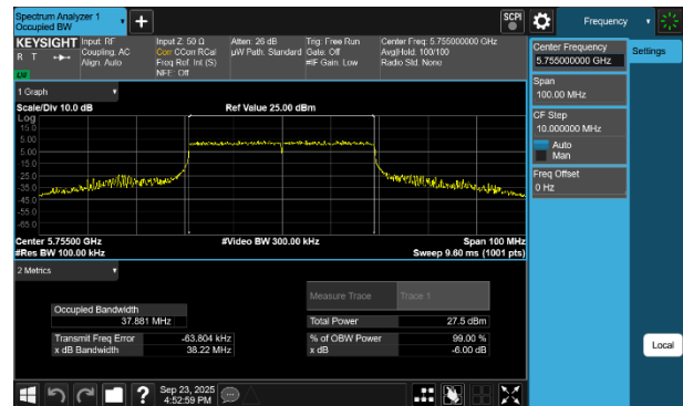
Plot 7-56 6dB OBW Antenna WF7b (40MHz BW 802.11be(RU) RU484 Index65 - Ch.151)
