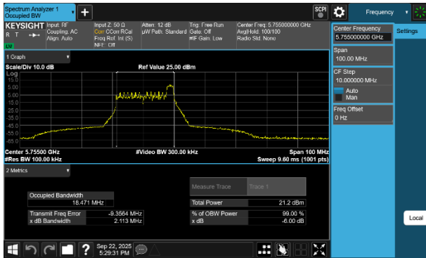
Plot 7-43 6dB OBW Antenna WF2a (40MHz BW 802.11be(RU) RU26 Index8 - Ch.151)
