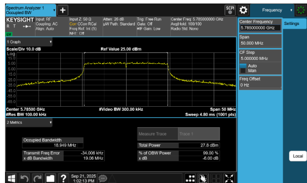
Plot 7-39 6dB OBW Antenna WF7a (20MHz BW 802.11be(RU) RU242 Index61 - Ch.157)
