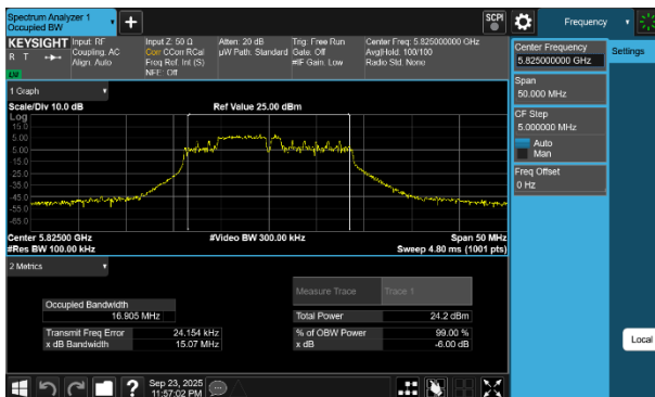
Plot 7-53 6dB OBW Antenna WF7b (20MHz BW 802.11be(RU) RU52+26 Index71 - Ch.165)
