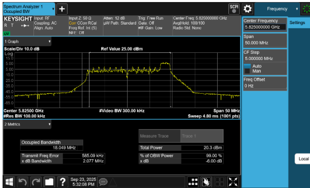
Plot 7-50 6dB OBW Antenna WF7b (20MHz BW 802.11be(RU) RU26 Index8 - Ch.165)
