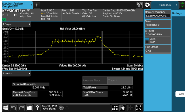
Plot 7-42 6dB OBW Antenna WF2a (20MHz BW 802.11be(RU) RU26 Index8 - Ch.165)
