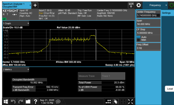
Plot 7-34 6dB OBW Antenna WF7a (20MHz BW 802.11be(RU) RU26 Index8 - Ch.149)
