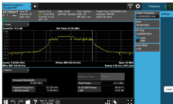
Plot 7-37 6dB OBW Antenna WF7a (20MHz BW 802.11be(RU) RU52+26 Index71 - Ch.165)
