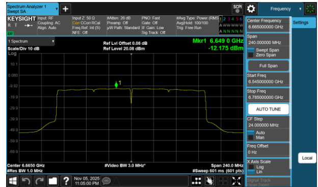
Plot 7-60 PSD Antenna 5T (160MHz BW 802.11be(SU) - Ch.143)
