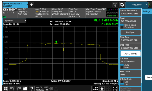
Plot 7-56 PSD Antenna 5T (160MHz BW 802.11be(SU) - Ch.111)
