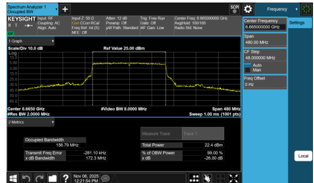
Plot 7-28 26dB BW & 99% OBW Antenna 3b (160MHz BW 802.11be(SU) - Ch.143)
