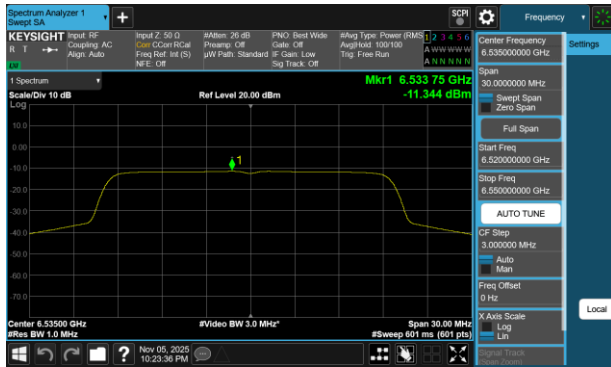
Plot 7-57 PSD Antenna 5T (20MHz BW 802.11be(SU) - Ch.117)
