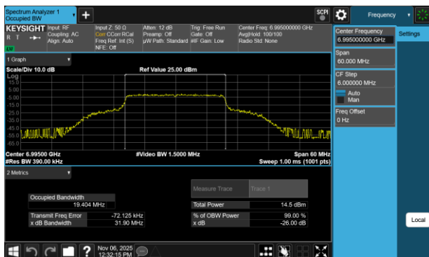
Plot 7-29 26dB BW & 99% OBW Antenna 3b (20MHz BW 802.11be(SU) - Ch.209)
