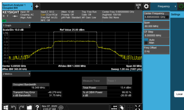
Plot 7-41 26dB BW & 99% OBW Antenna 1b (20MHz BW 802.11be(SU) - Ch.149)
