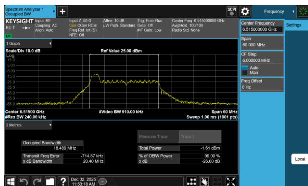
Plot 7-56 26dB BW & 99% OBW Antenna 3b (20MHz BW 802.11be(RU) RU26 Index0 - Ch.113)
