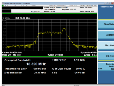
Plot 7-56 26dB BW & 99% OBW Antenna 5T (20MHz BW 802.11be(RU) RU26 Index8 - Ch.149)
