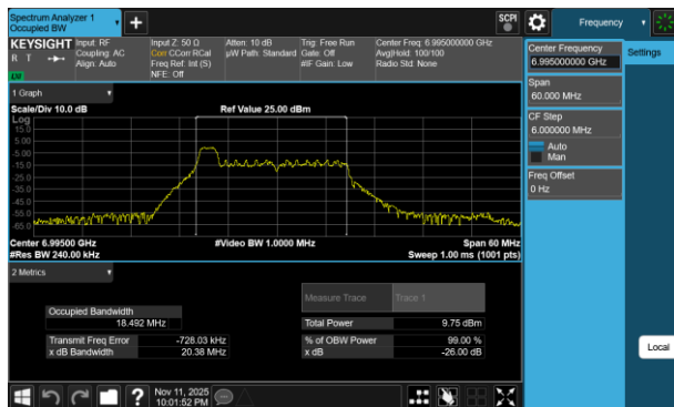
Plot 7-144 26dB BW & 99% OBW Antenna 3b (20MHz BW 802.11be(RU) RU26 Index0 - Ch.209)
