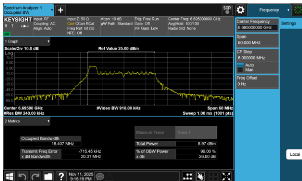
Plot 7-133 26dB BW & 99% OBW Antenna 3b (20MHz BW 802.11be(RU) RU26 Index0 - Ch.149)
