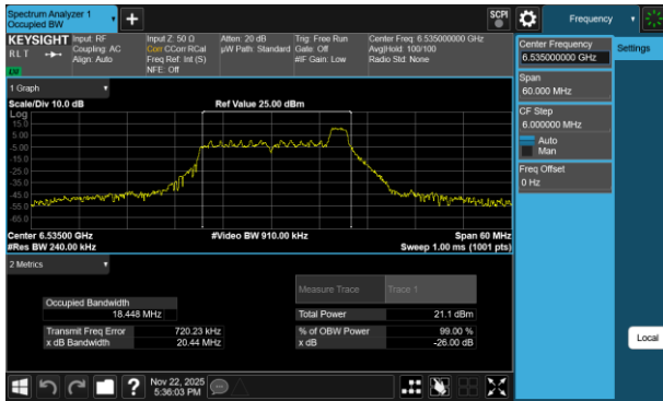
Plot 7-177 26dB BW & 99% OBW Antenna 1b (20MHz BW 802.11be(RU) RU26 Index8 - Ch.117)
