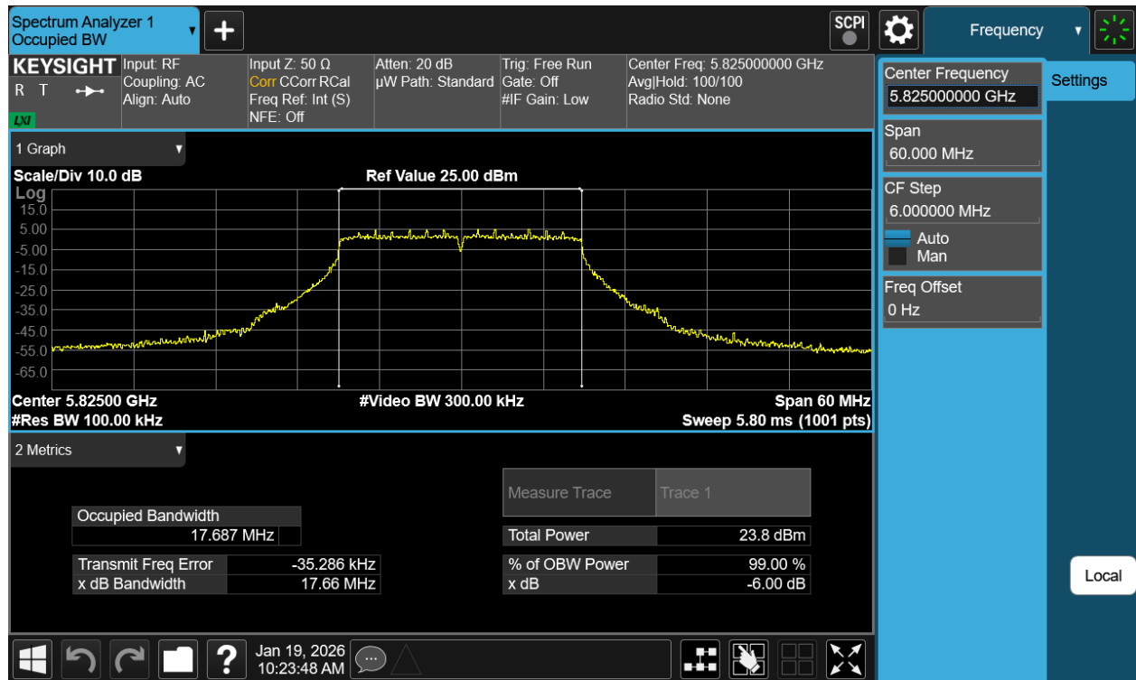
Plot 7-16 6dB OBW Antenna 3b (20MHz BW 802.11a - Ch.165)
