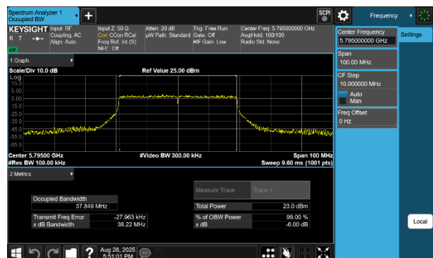
Plot 7-48 6dB OBW Antenna 3b (40MHz BW 802.11be(RU) RU484 Index65 - Ch.159)
