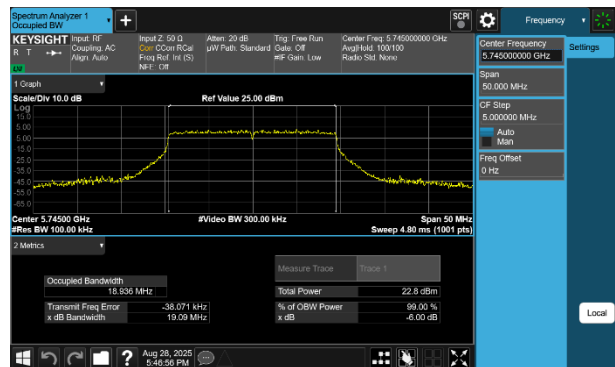
Plot 7-47 6dB OBW Antenna 3b (20MHz BW 802.11be(RU) RU242 Index61 - Ch.149)
