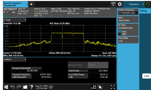
Plot 7-54 6dB OBW Antenna 1b (80MHz BW 802.11be(RU) RU484+242 Index90 - Ch.155)
