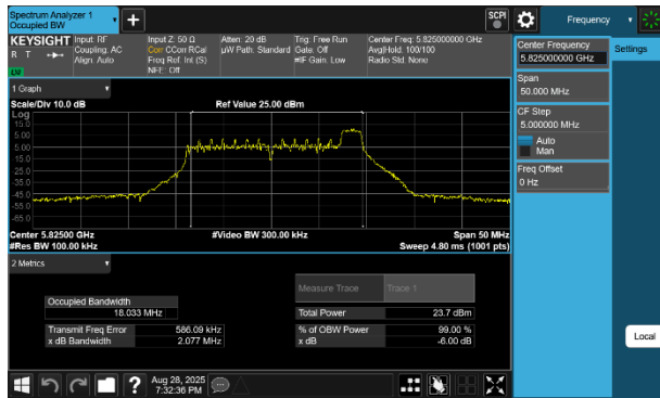
Plot 7-42 6dB OBW Antenna 3b (20MHz BW 802.11be(RU) RU26 Index8 - Ch.165)
