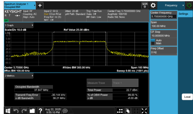
Plot 7-56 6dB OBW Antenna 1b (40MHz BW 802.11be(RU) RU484 Index65 - Ch.151)
