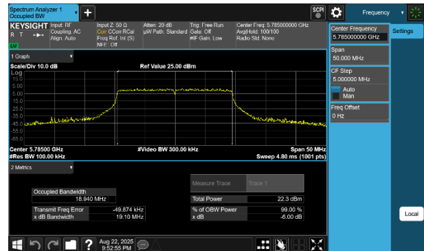
Plot 7-55 6dB OBW Antenna 1b (20MHz BW 802.11be(RU) RU242 Index61 - Ch.157)
