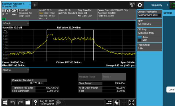
Plot 7-50 6dB OBW Antenna 1b (20MHz BW 802.11be(RU) RU26 Index0 - Ch.165)
