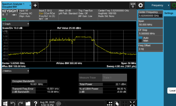
Plot 7-53 6dB OBW Antenna 1b (20MHz BW 802.11be(RU) RU52+26 Index72 - Ch.165)
