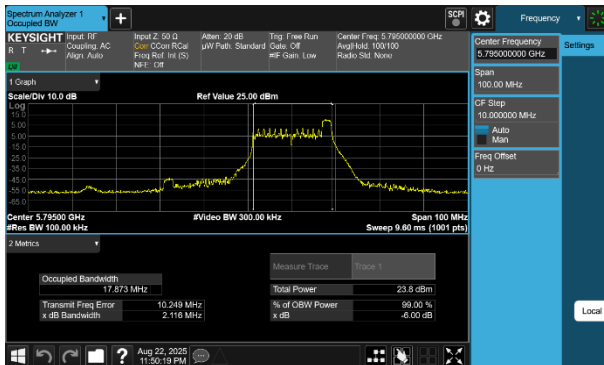
Plot 7-51 6dB OBW Antenna 1b (40MHz BW 802.11be(RU) RU26 Index17 - Ch.159)
