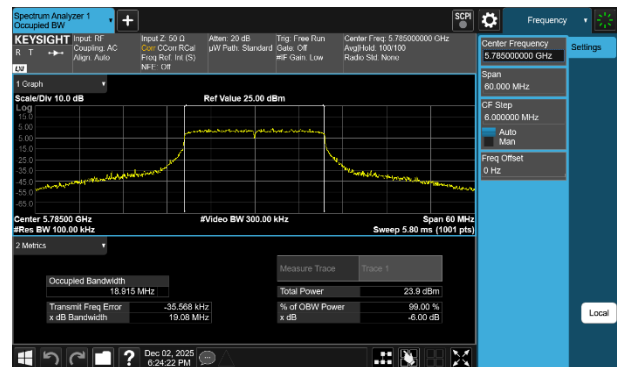
Plot 7-39 6dB OBW Antenna 5T (20MHz BW 802.11be(RU) RU242 Index61 - Ch.157)
