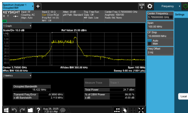
Plot 7-43 6dB OBW Antenna 3b (40MHz BW 802.11be(RU) RU26 Index8 - Ch.159)
