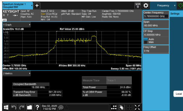
Plot 7-34 6dB OBW Antenna 5T (20MHz BW 802.11be(RU) RU26 Index8 - Ch.157)
