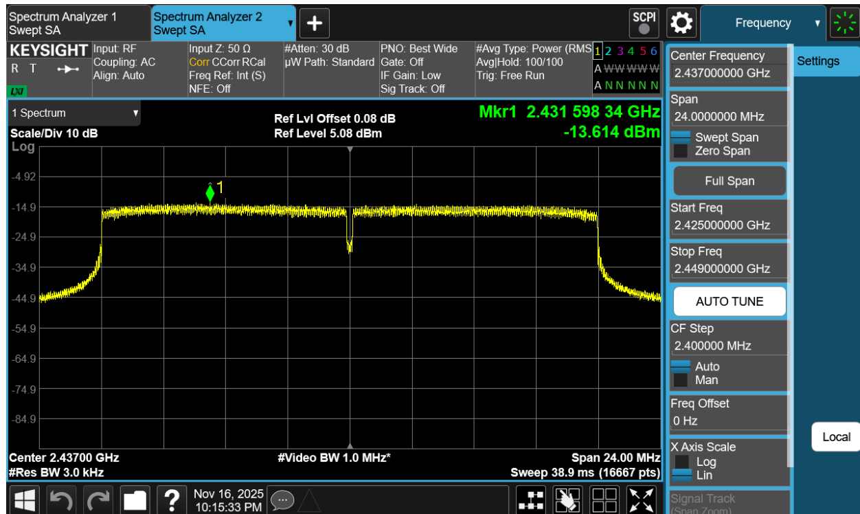
Plot 7-20 PSD Antenna 3a (20MHz BW 802.11be(SU) - Ch.6)
