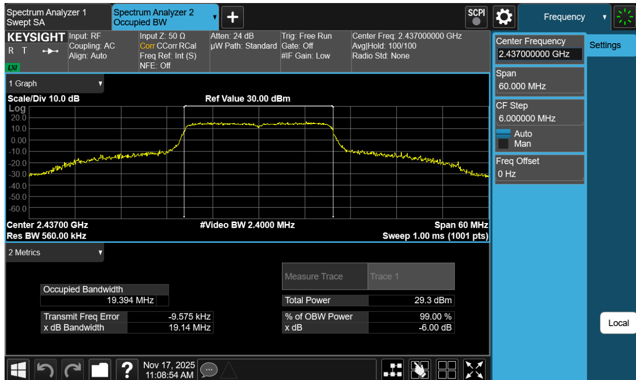
Plot 7-8 99% OBW Antenna 1a (20MHz BW 802.11be(SU) - Ch.6)
