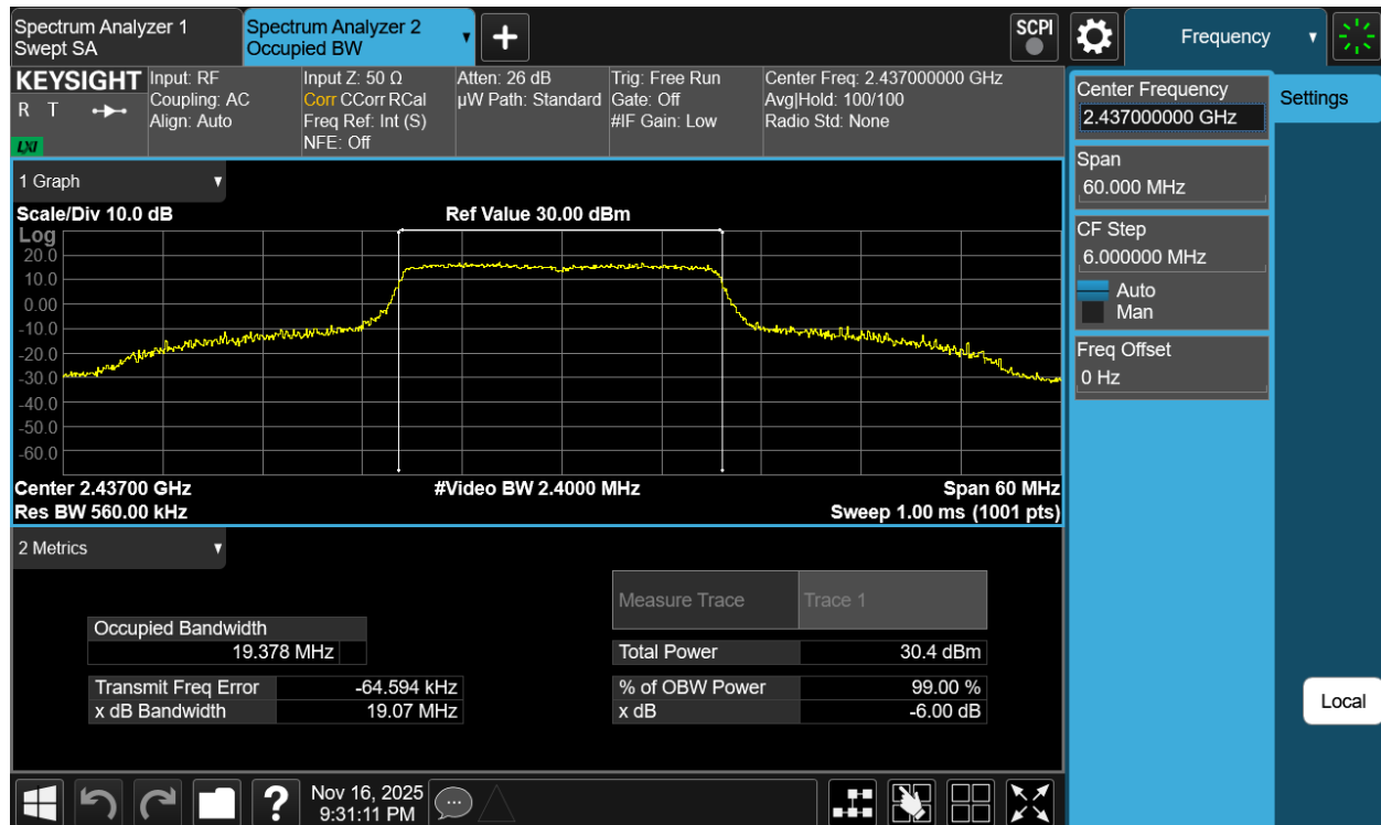
Plot 7-4 99% OBW Antenna 3a (20MHz BW 802.11be(SU) - Ch.6)
