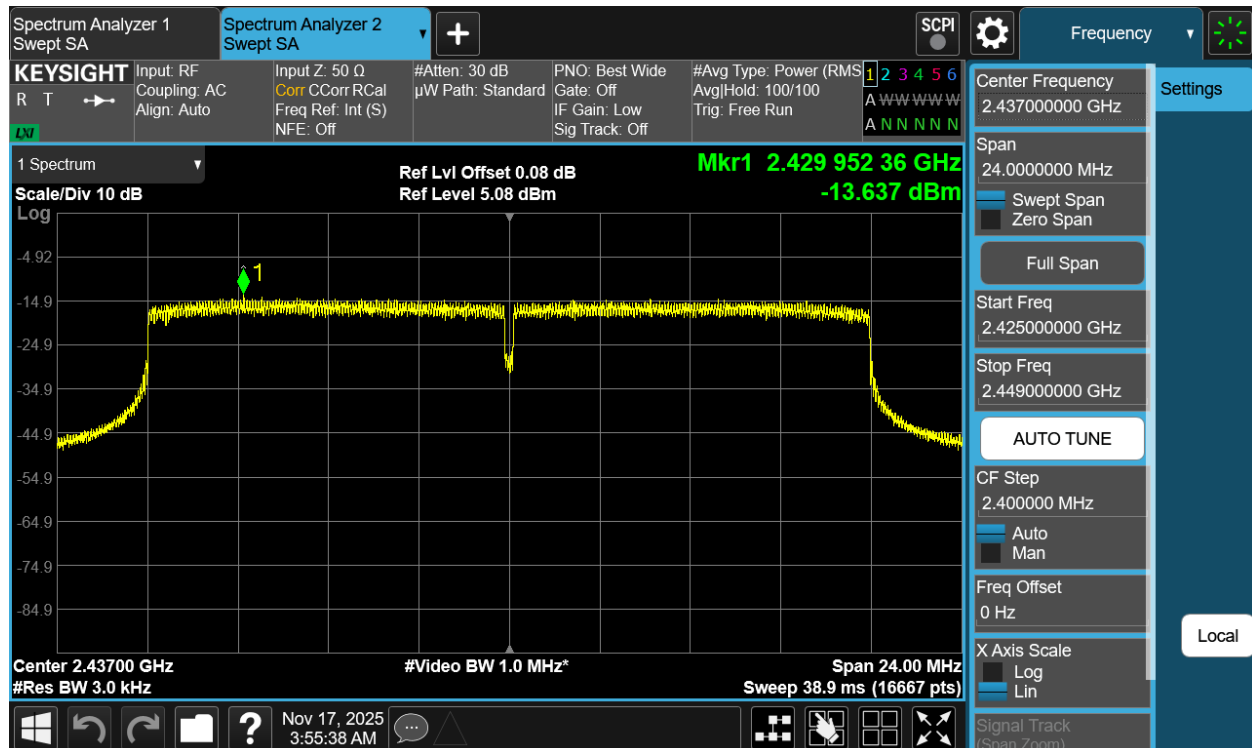
Plot 7-28 PSD CDD Antenna 3a (20MHz BW 802.11be(SU) - Ch.6)
