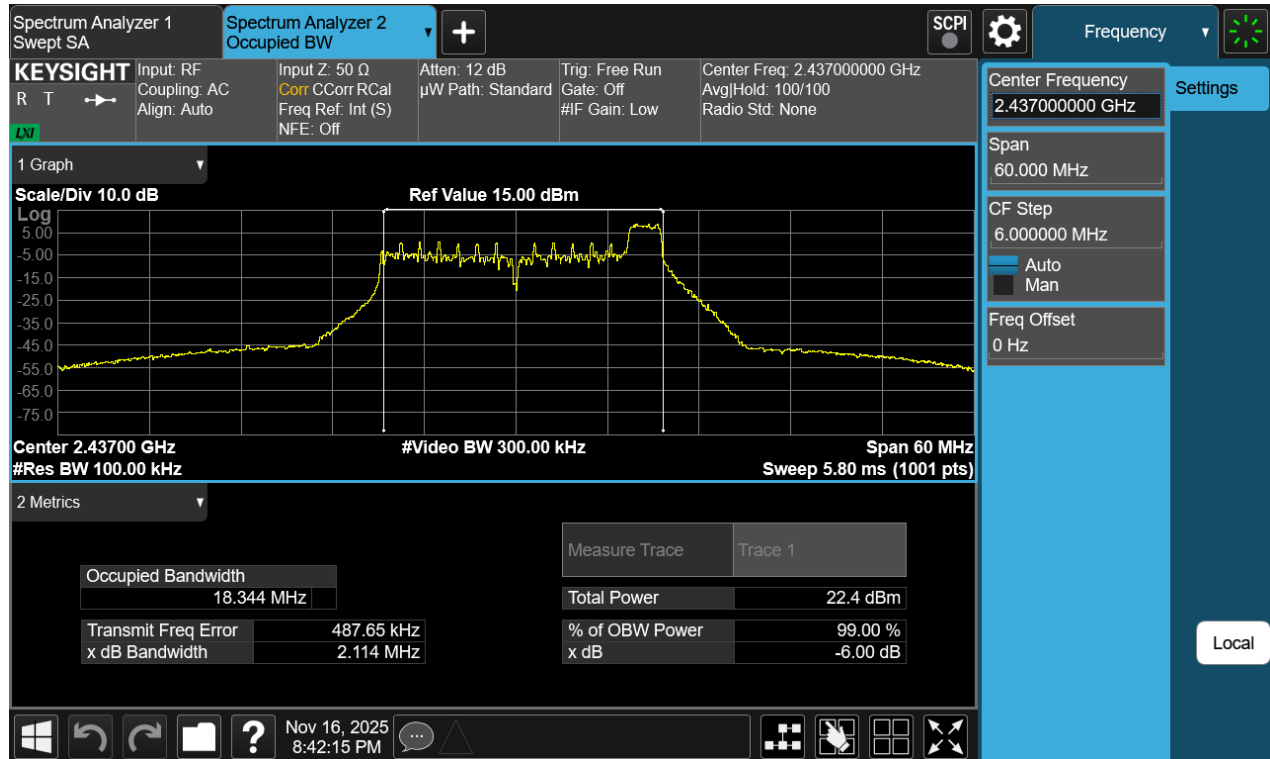
Plot 7-9 6dB OBW Antenna 3a (20MHz BW 802.11be(RU) RU26 Index8 - Ch.6)
