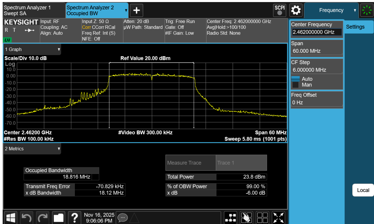
Plot 7-10 6dB OBW Antenna 3a (20MHz BW 802.11be(RU) RU242 Index61 - Ch.11)
