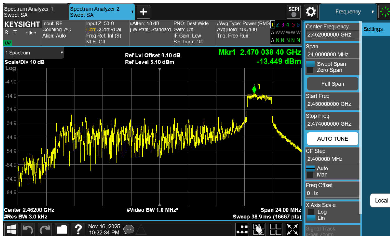
Plot 7-17 PSD Antenna 3a (20MHz BW 802.11be(RU) RU26 Index8 - Ch.11)
