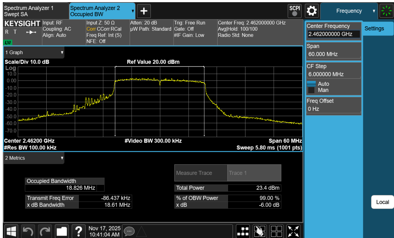
Plot 7-14 6dB OBW Antenna 1a (20MHz BW 802.11be(RU) RU242 Index61 - Ch.11)
