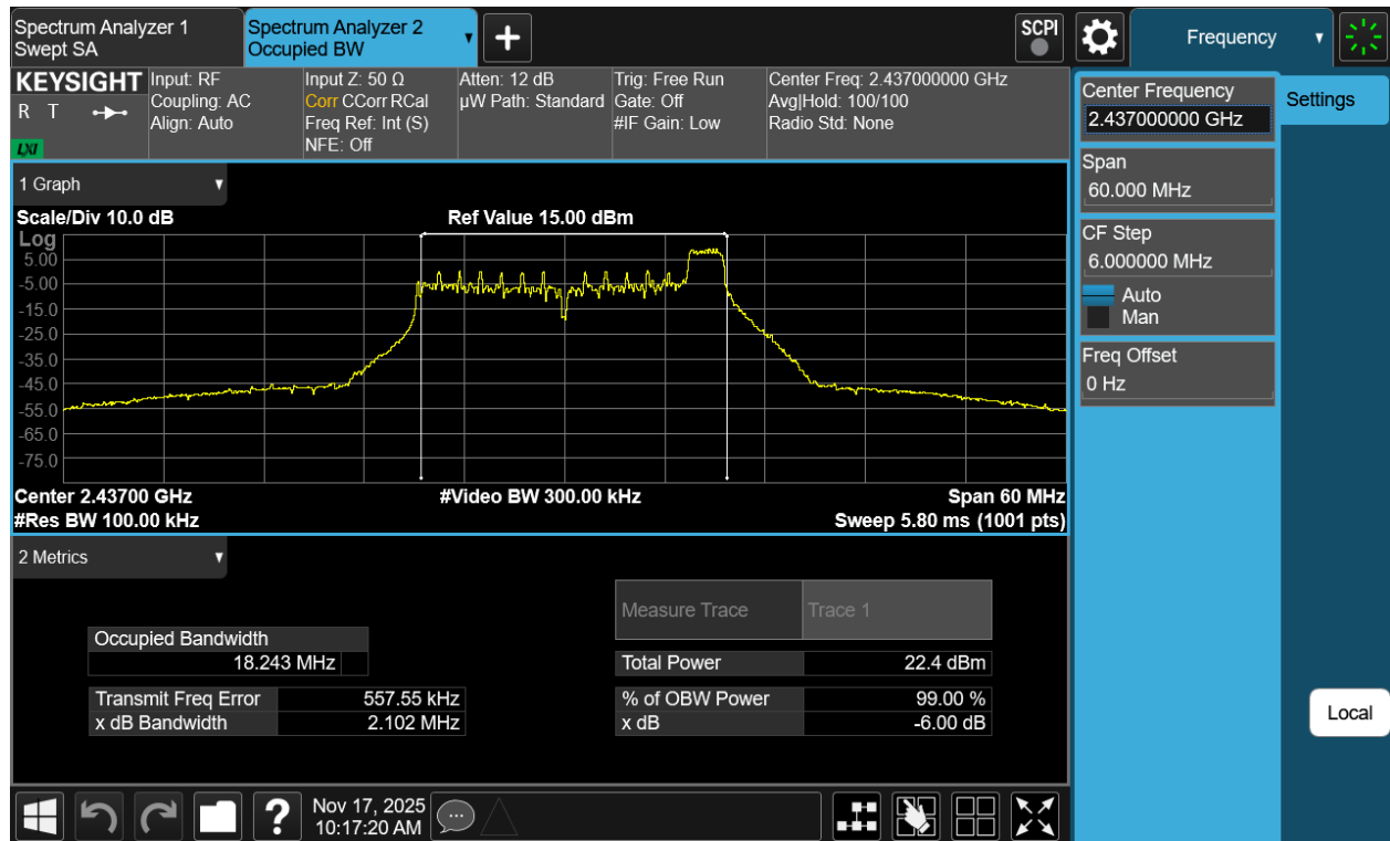
Plot 7-13 6dB OBW Antenna 1a (20MHz BW 802.11be(RU) RU26 Index8 - Ch.6)
