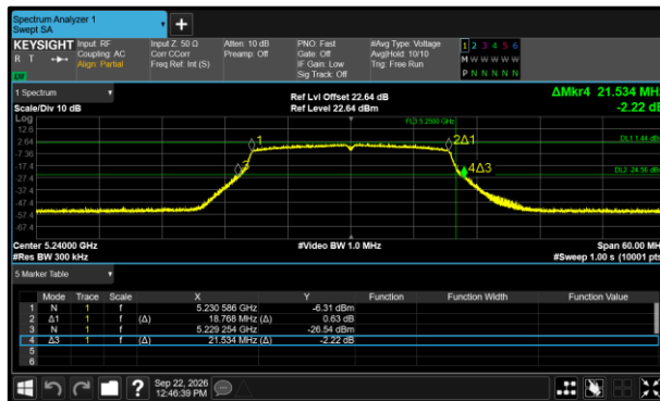
Figure 381 - 802.11ax HE20 SU Minimum 99% OBW
