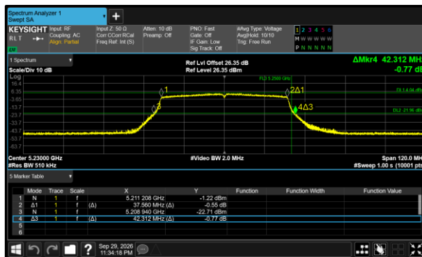
Figure 383 - 802.11ax HE40 SU Minimum 99% OBW
