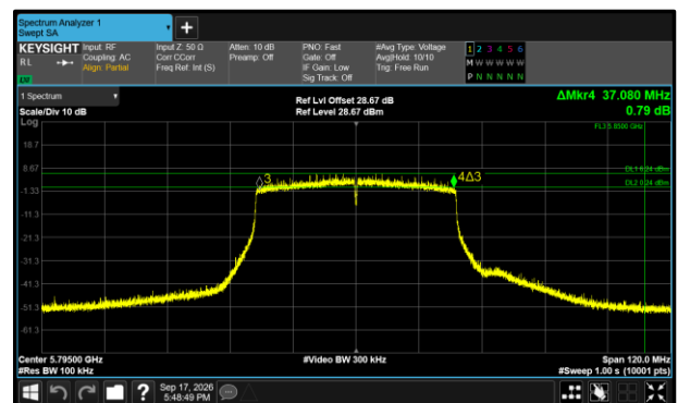
Figure 434 - 802.11ax HE40 SU Maximum 6 dB EBW
