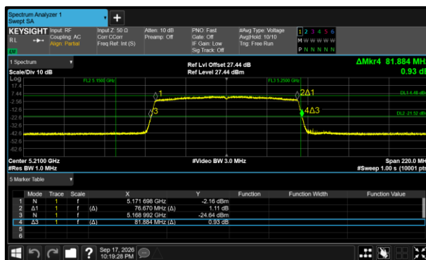
Figure 401 - 802.11ax HE80 SU Minimum 99% OBW
