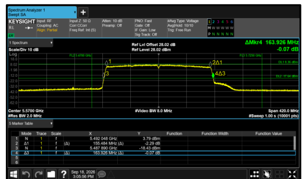
Figure 364 - 802.11ax HE160 SU Maximum 99% OBW
