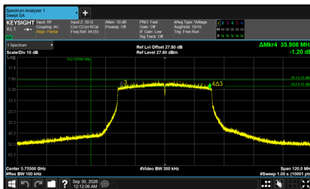
Figure 421 - 802.11ax HE40 SU Minimum 6 dB EBW
