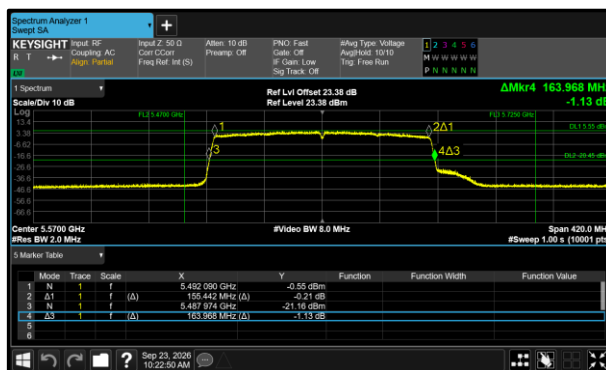
Figure 387 - 802.11ax HE160 SU Minimum 99% OBW
