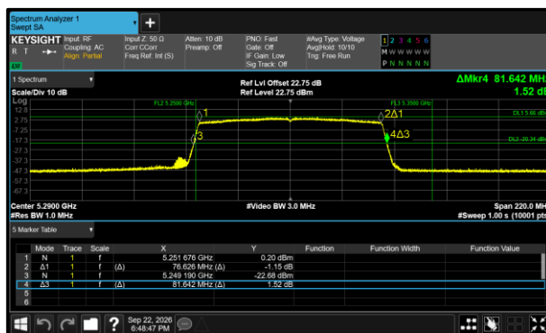
Figure 385 - 802.11ax HE80 SU Minimum 99% OBW
