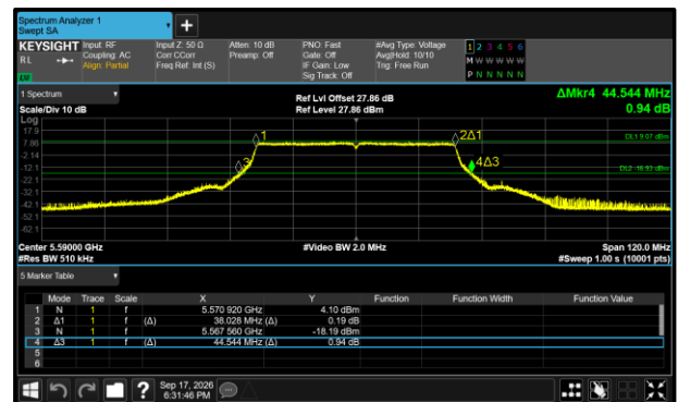
Figure 400 - 802.11ax HE40 SU Maximum 99% OBW
