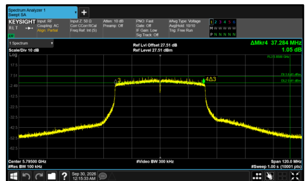
Figure 422 - 802.11ax HE40 SU Maximum 6 dB EBW
