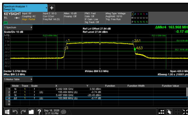
Figure 403 - 802.11ax HE160 SU Minimum 99% OBW
