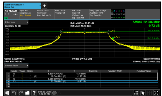
Figure 382 - 802.11ax HE20 SU Maximum 99% OBW
