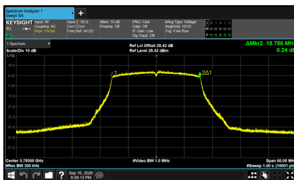
Figure 357 - 802.11ax HE20 SU Minimum 99% OBW
