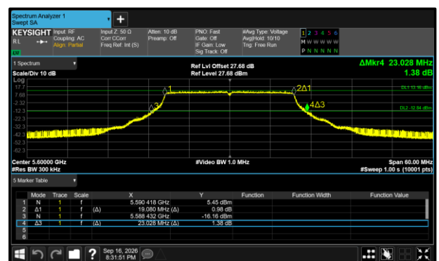
Figure 358 - 802.11ax HE20 SU Maximum 99% OBW
