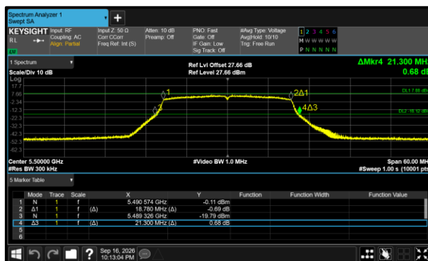
Figure 397 - 802.11ax HE20 SU Minimum 99% OBW
