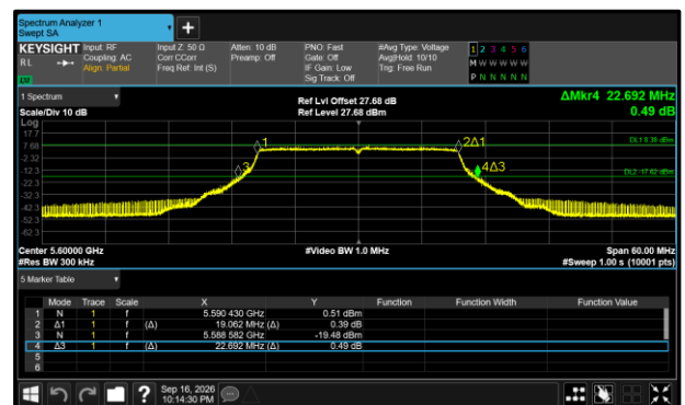
Figure 398 - 802.11ax HE20 SU Maximum 99% OBW
