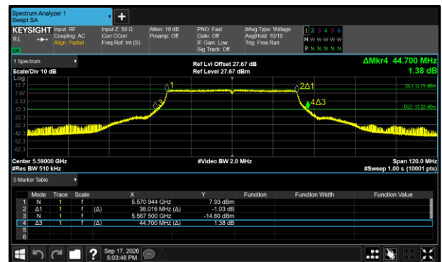
Figure 360 - 802.11ax HE40 SU Maximum 99% OBW
