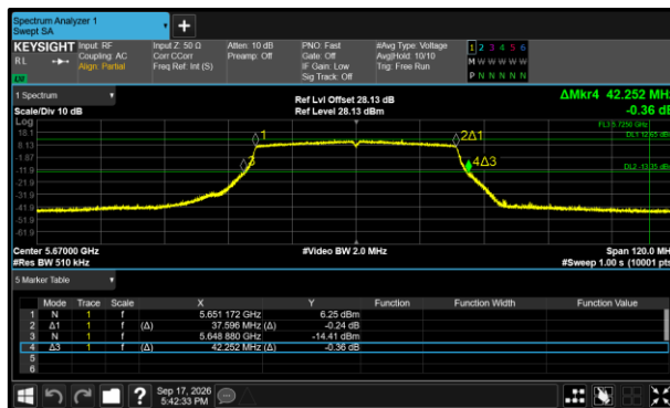
Figure 359 - 802.11ax HE40 SU Minimum 99% OBW
