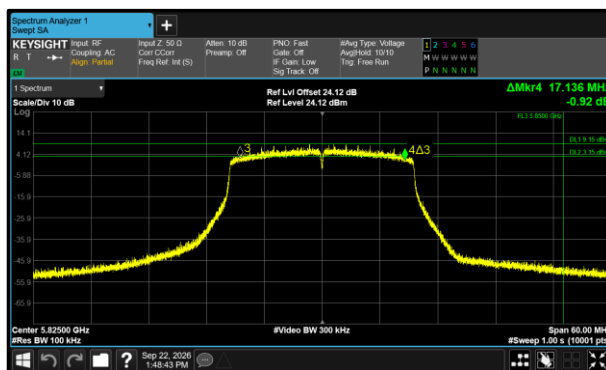
Figure 419 - 802.11ax HE20 SU Minimum 6 dB EBW
