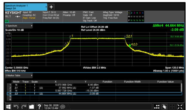
Figure 384 - 802.11ax HE40 SU Maximum 99% OBW
