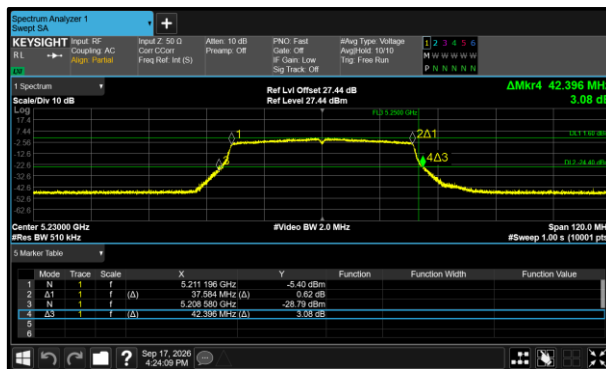
Figure 399 - 802.11ax HE40 SU Minimum 99% OBW
