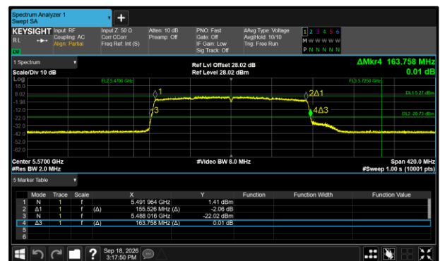
Figure 404 - 802.11ax HE160 SU Maximum 99% OBW
