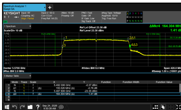
Figure 347 - 802.11ax HE160 SU Minimum 99% OBW
