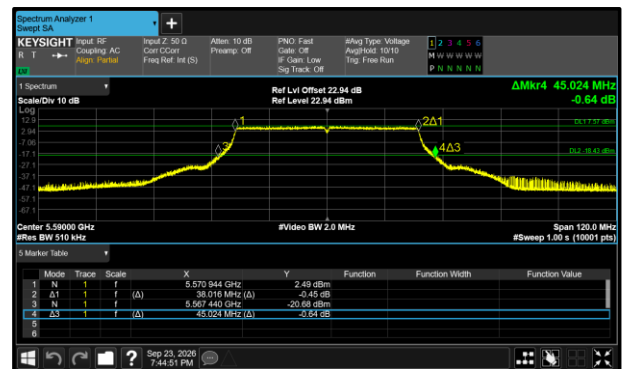
Figure 328 - 802.11ax HE40 SU Maximum 26 dB EBW
