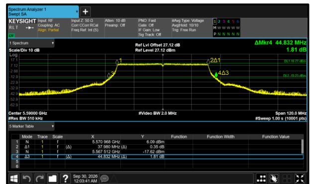
Figure 288 - 802.11ax HE40 SU Maximum 26 dB EBW
