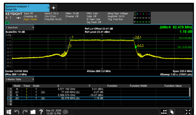
Figure 346 - 802.11ax HE80 SU Maximum 99% OBW
