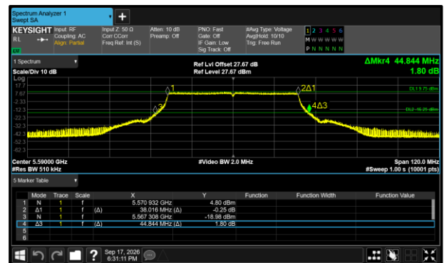
Figure 304 - 802.11ax HE40 SU Maximum 26 dB EBW
