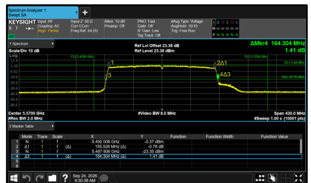
Figure 348 - 802.11ax HE160 SU Maximum 99% OBW
