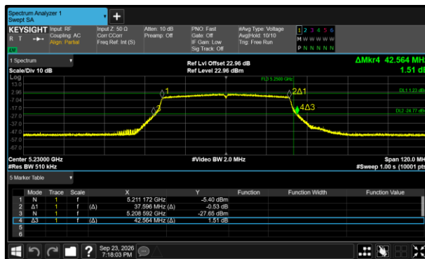
Figure 343 - 802.11ax HE40 SU Minimum 99% OBW
