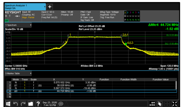
Figure 344 - 802.11ax HE40 SU Maximum 99% OBW
