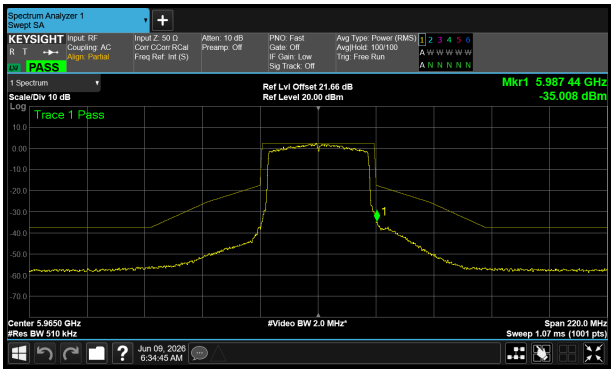
5965 MHz – Core 1
