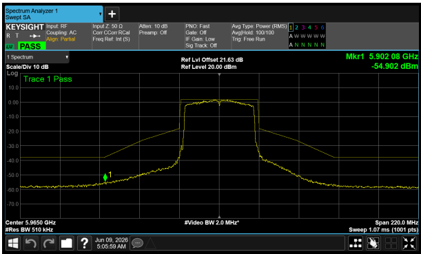
5965 MHz – Core 0
