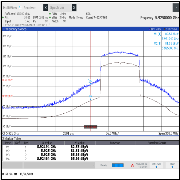
Lower Band Edge / Channel 7
