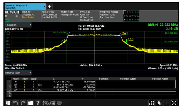
Figure 258 - 802.11ax HE20 SU VLP Maximum 99% OBW
