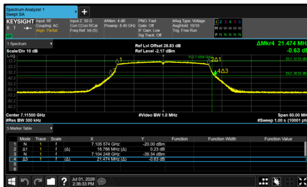
Figure 257 - 802.11ax HE20 SU VLP Minimum 99% OBW
