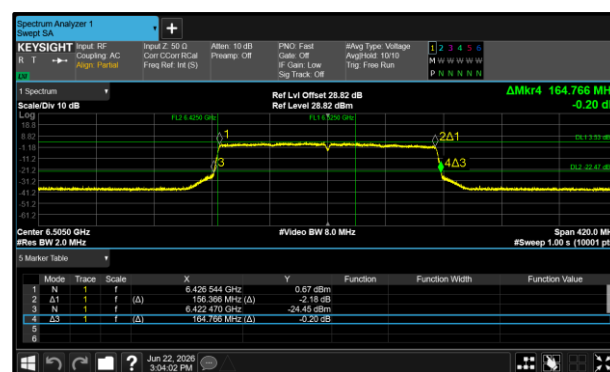
Figure 248 - 802.11ax HE160 SU LPI Maximum 99% OBW
