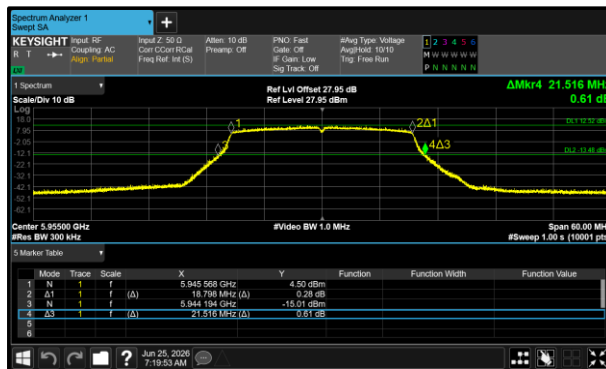
Figure 249 - 802.11ax HE20 SU SP Minimum 99% OBW
