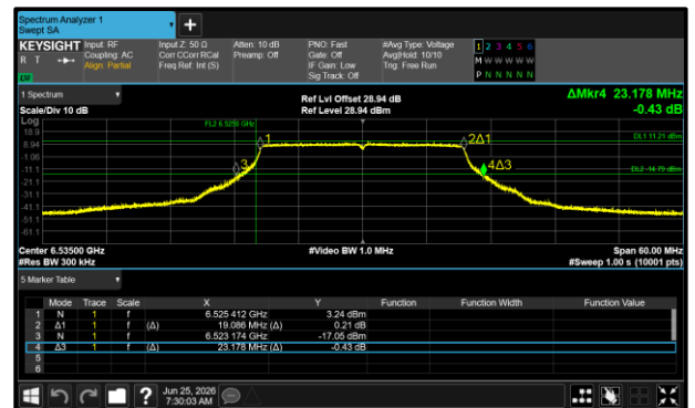
Figure 250 - 802.11ax HE20 SU SP Maximum 99% OBW
