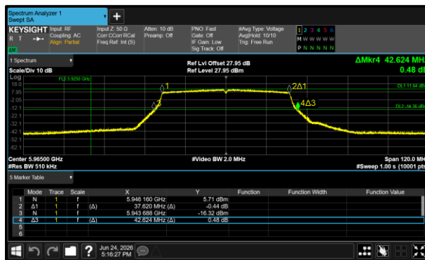
Figure 251 - 802.11ax HE40 SU SP Minimum 99% OBW
