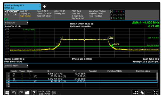
Figure 260 - 802.11ax HE40 SU VLP Maximum 99% OBW
