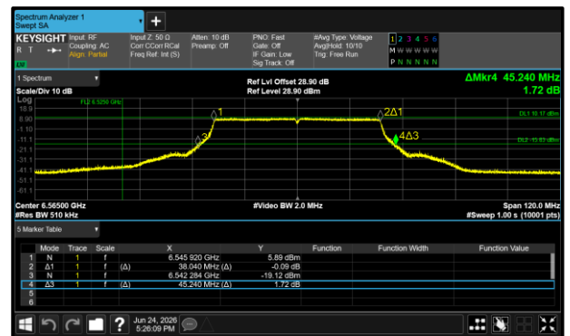
Figure 252 - 802.11ax HE40 SU SP Maximum 99% OBW
