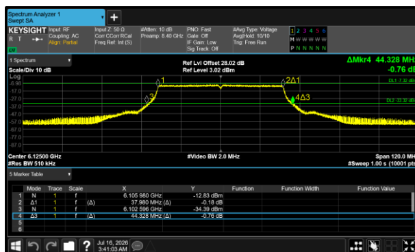
Figure 259 - 802.11ax HE40 SU VLP Minimum 99% OBW
