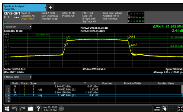
Figure 253 - 802.11ax HE80 SU SP Minimum 99% OBW
