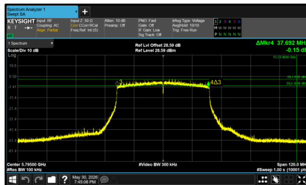
Figure 100 - 802.11ax HE40 SU Maximum 6 dB EBW
