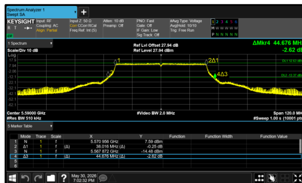
Figure 12 - 802.11ax HE40 SU Maximum 26 dB EBW
