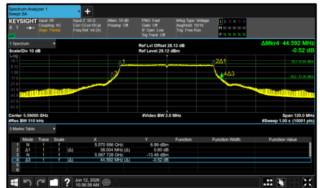
Figure 12 - 802.11ax HE40 SU Maximum 26 dB EBW
