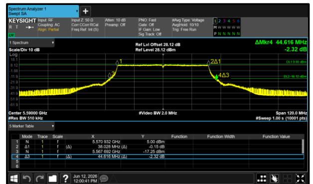
Figure 186 - 802.11ax HE40 SU Maximum 99% OBW
