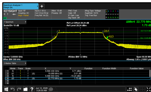
Figure 118 - 802.11ax HE20 SU Maximum 99% OBW
