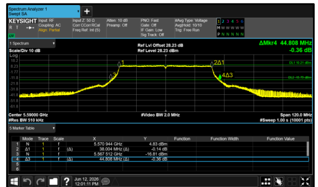
Figure 144 - 802.11ax HE40 SU Maximum 26 dB EBW
