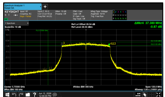
Figure 166 - 802.11ax HE40 SU Maximum 6 dB EBW
