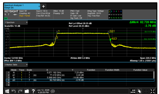
Figure 122 - 802.11ax HE80 SU Maximum 99% OBW
