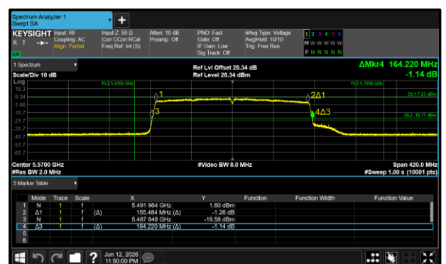
Figure 124 - 802.11ax HE160 SU Maximum 99% OBW
