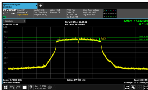
Figure 163 - 802.11ax HE20 SU Minimum 6 dB EBW
