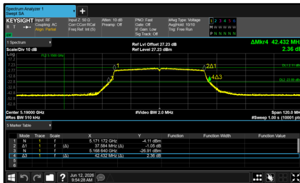
Figure 185 - 802.11ax HE40 SU Minimum 99% OBW
