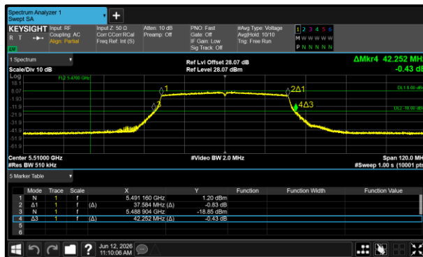
Figure 119 - 802.11ax HE40 SU Minimum 99% OBW
