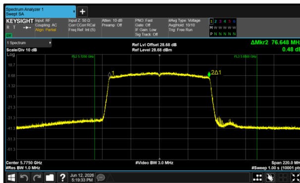
Figure 187 - 802.11ax HE80 SU Minimum 99% OBW
