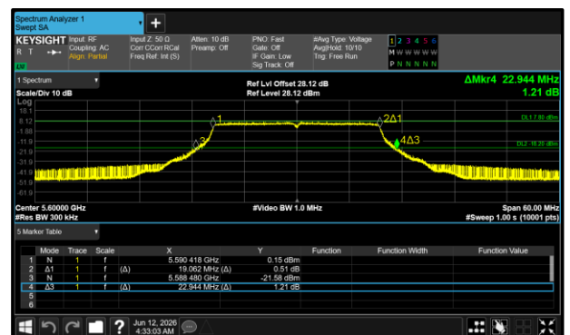
Figure 142 - 802.11ax HE20 SU Maximum 26 dB EBW
