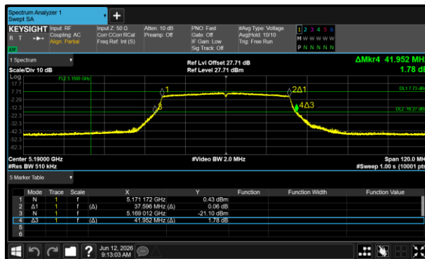
Figure 143 - 802.11ax HE40 SU Minimum 26 dB EBW
