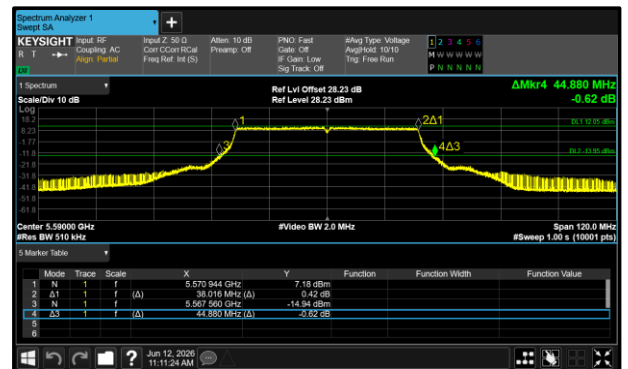
Figure 120 - 802.11ax HE40 SU Maximum 99% OBW
