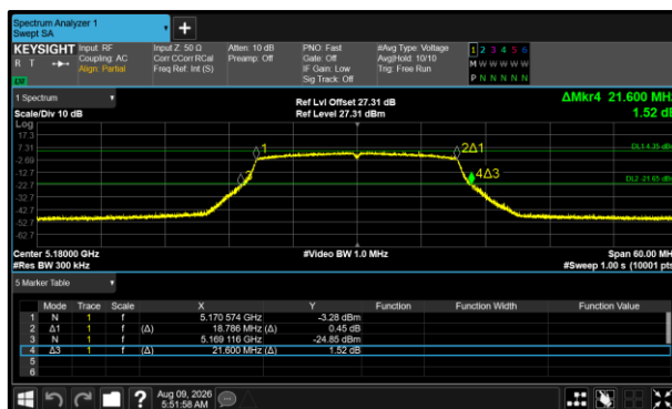
Figure 484 - 802.11ax HE20 SU Minimum 99% OBW
