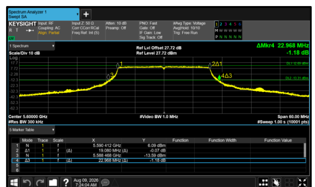
Figure 461 - 802.11ax HE20 SU Maximum 26 dB EBW
