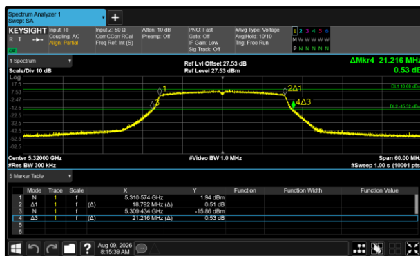
Figure 508 - 802.11ax HE20 SU Minimum 26 dB EBW
