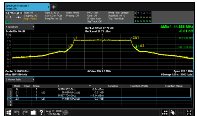
Figure 463 - 802.11ax HE40 SU Maximum 26 dB EBW
