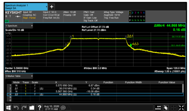
Figure 487 - 802.11ax HE40 SU Maximum 99% OBW
