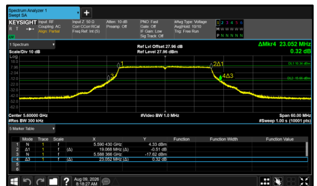
Figure 485 - 802.11ax HE20 SU Maximum 99% OBW
