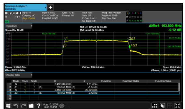
Figure 491 - 802.11ax HE160 SU Maximum 99% OBW
