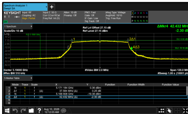
Figure 486 - 802.11ax HE40 SU Minimum 99% OBW
