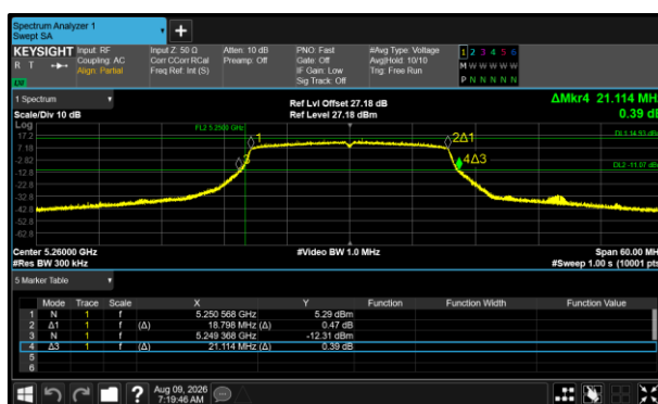
Figure 460 - 802.11ax HE20 SU Minimum 26 dB EBW
