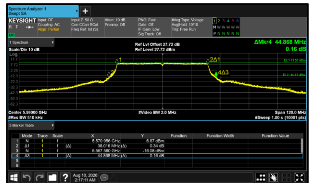
Figure 511 - 802.11ax HE40 SU Maximum 26 dB EBW
