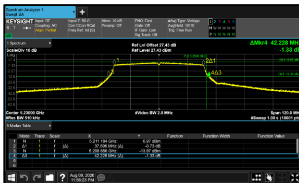
Figure 354 - 802.11ax HE40 SU Minimum 99% OBW
