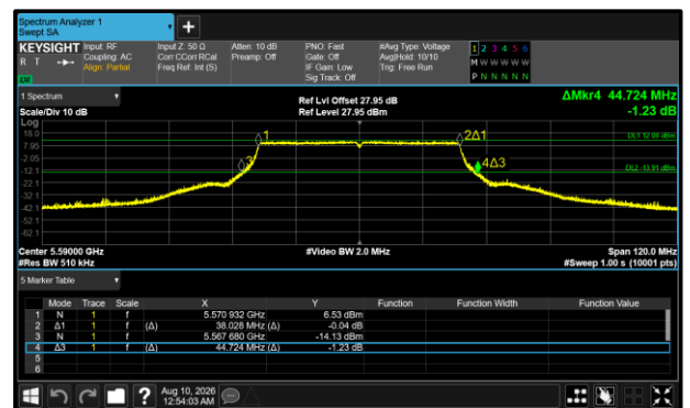
Figure 355 - 802.11ax HE40 SU Maximum 99% OBW
