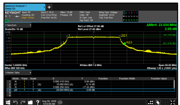
Figure 353 - 802.11ax HE20 SU Maximum 99% OBW
