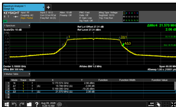
Figure 352 - 802.11ax HE20 SU Minimum 99% OBW
