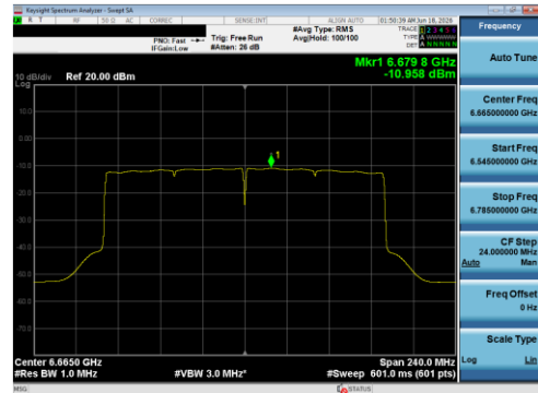
Plot 7-92 PSD Antenna 1B (160 MHz BW 802.11be(SU) - Ch.143)
