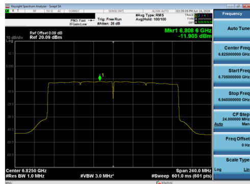
Plot 7-60 PSD Antenna 5T (160 MHz BW 802.11be(SU) - Ch.175)
