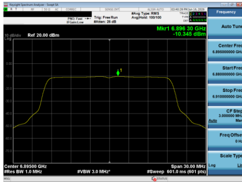
Plot 7-61 PSD Antenna 5T (20 MHz BW 802.11be(SU) - Ch.189)
