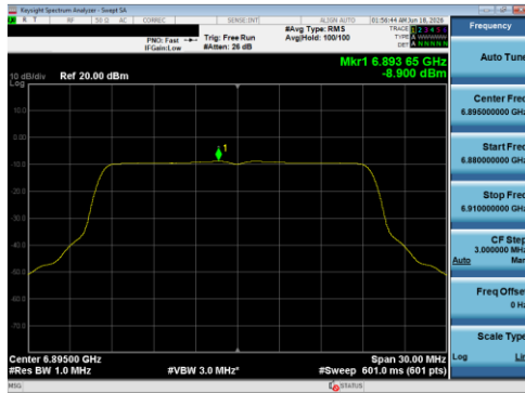
Plot 7-93 PSD Antenna 1B (20 MHz BW 802.11be(SU) - Ch.189)
