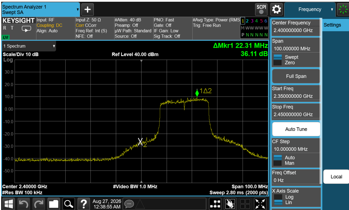
Plot 7-66. Band Edge Plot Antenna 3A (802.11be (SU - 2.4 GHz) – Ch. 2)
