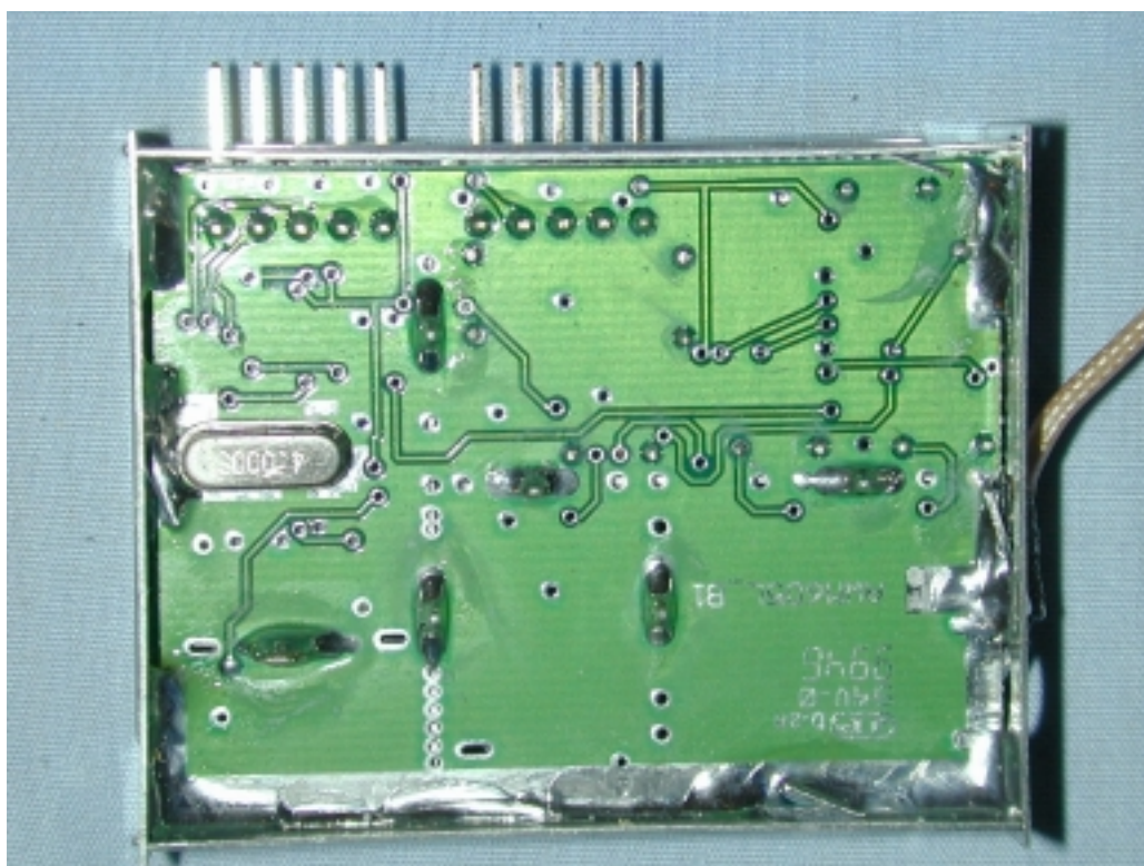
(20) EUT Photo
