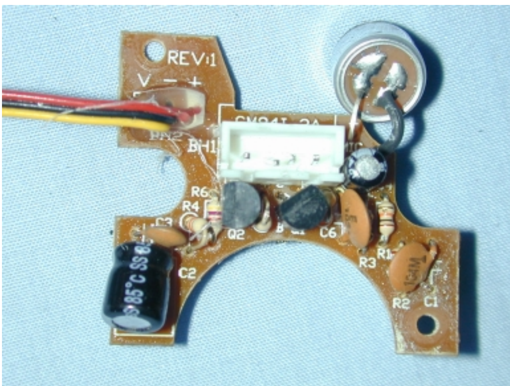
(12) EUT Photo
