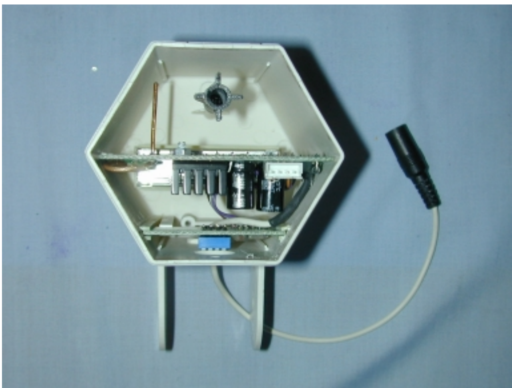
(14) EUT Photo
