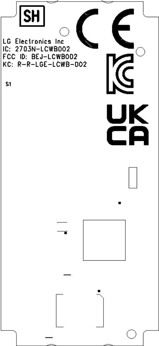
Bottom side
