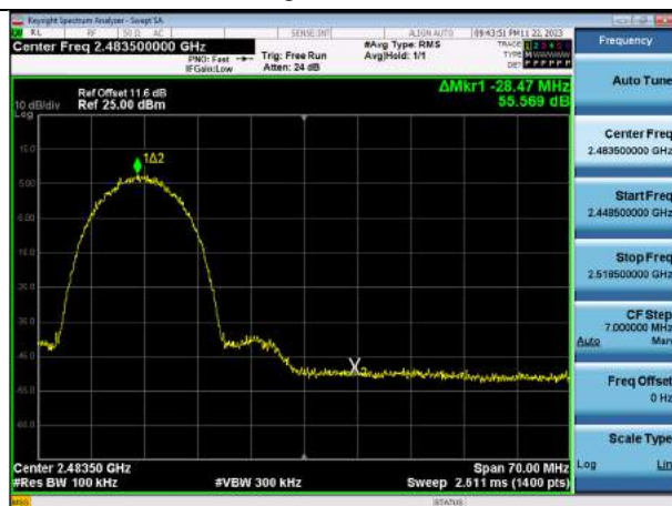
Band Edge (802.11g-CH11)
