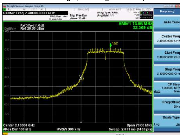
Band Edge (802.11n_HT20-CH1)
