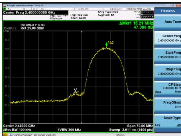
Band Edge (802.11g-CH1)
