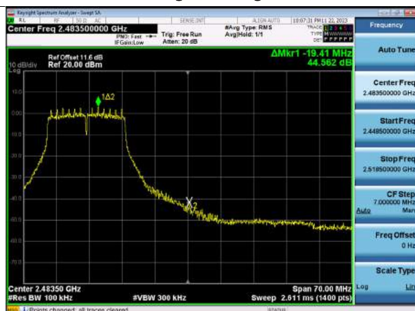
Band Edge (802.11n_HT20-CH11)
