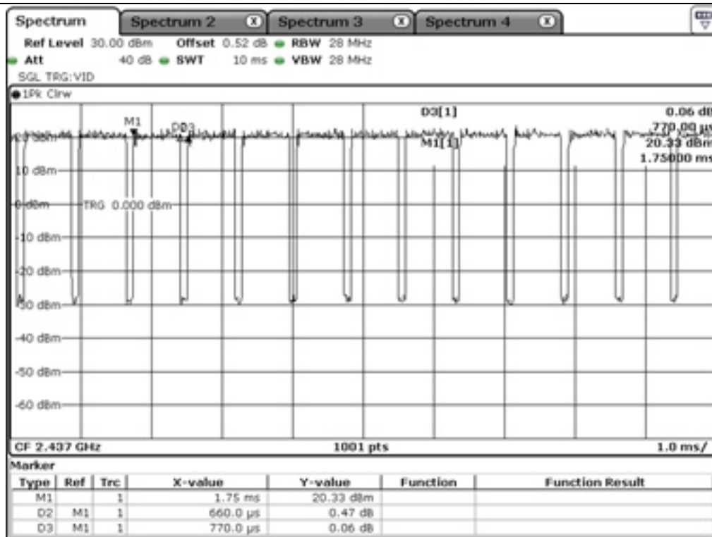
802.11 HT 20_Antenna 1
