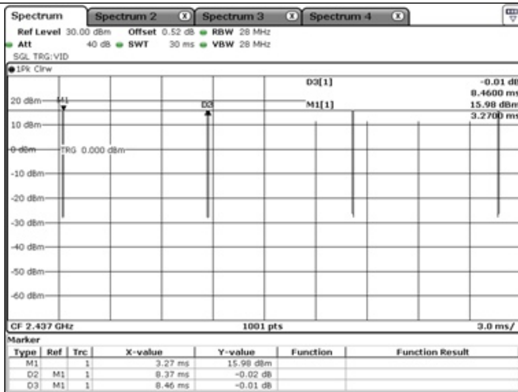
802.11 b_Antenna 1
