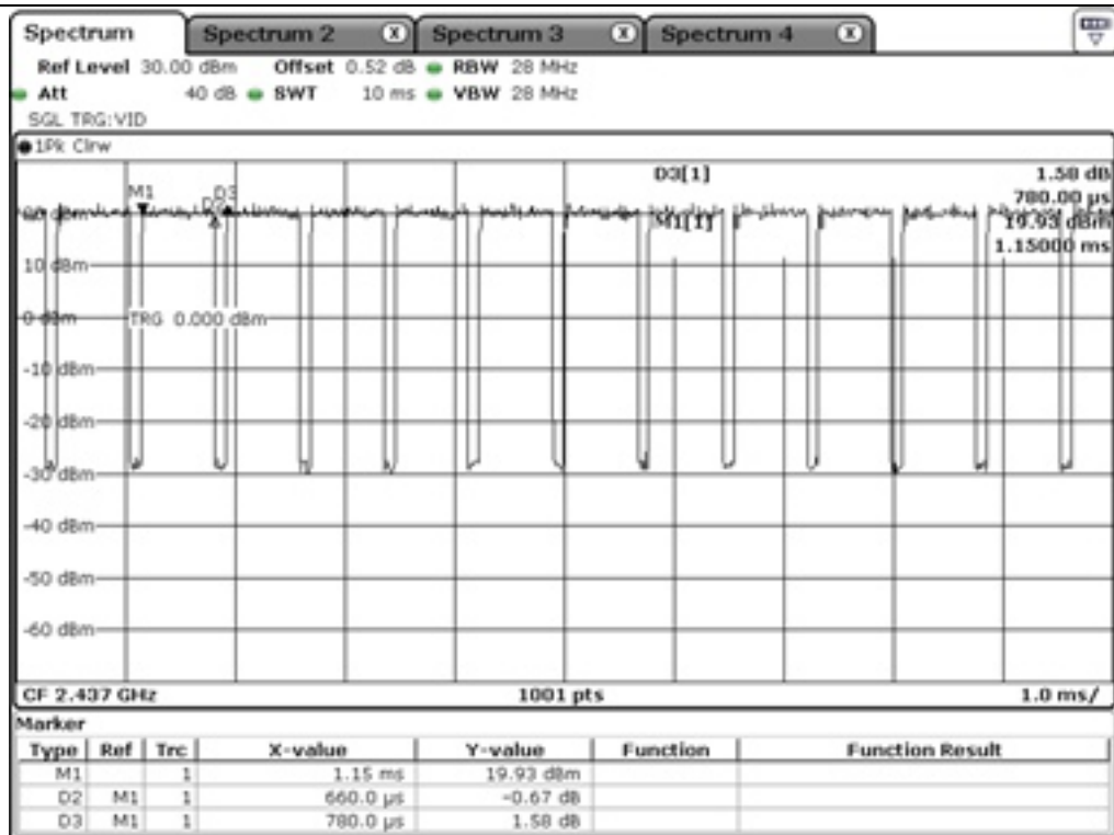
802.11 HT 20_Antenna 0
