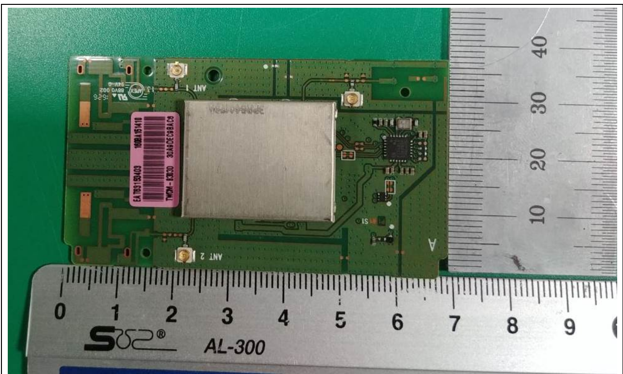
<WIFI Module>
