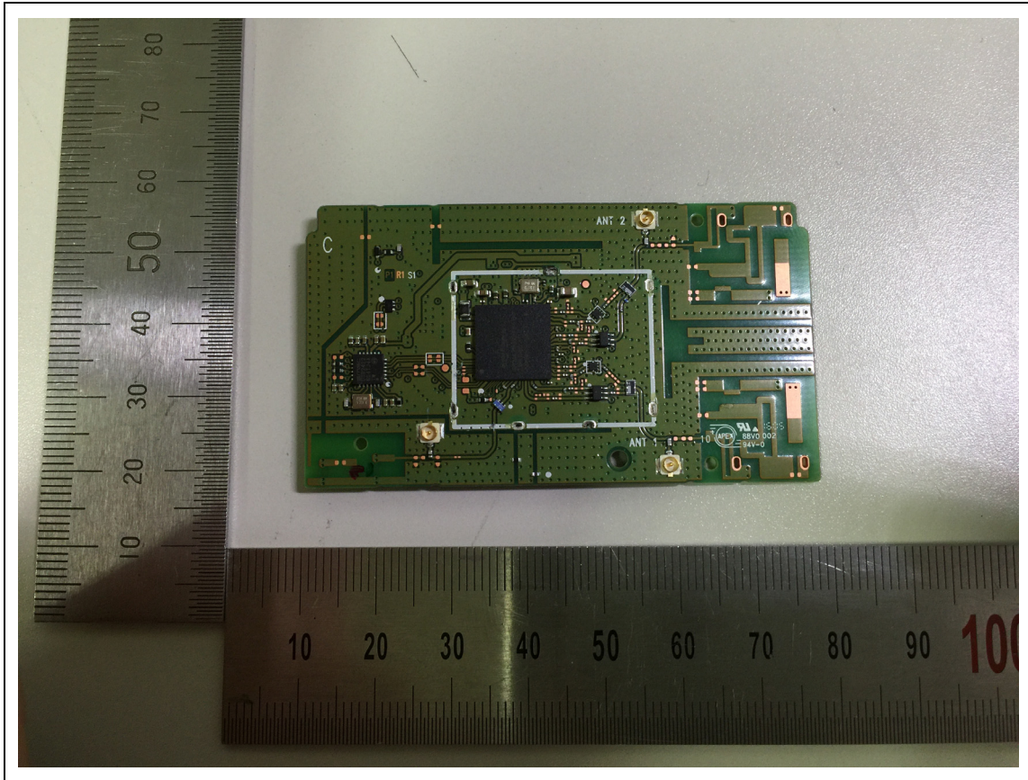
<WIFI Module>
