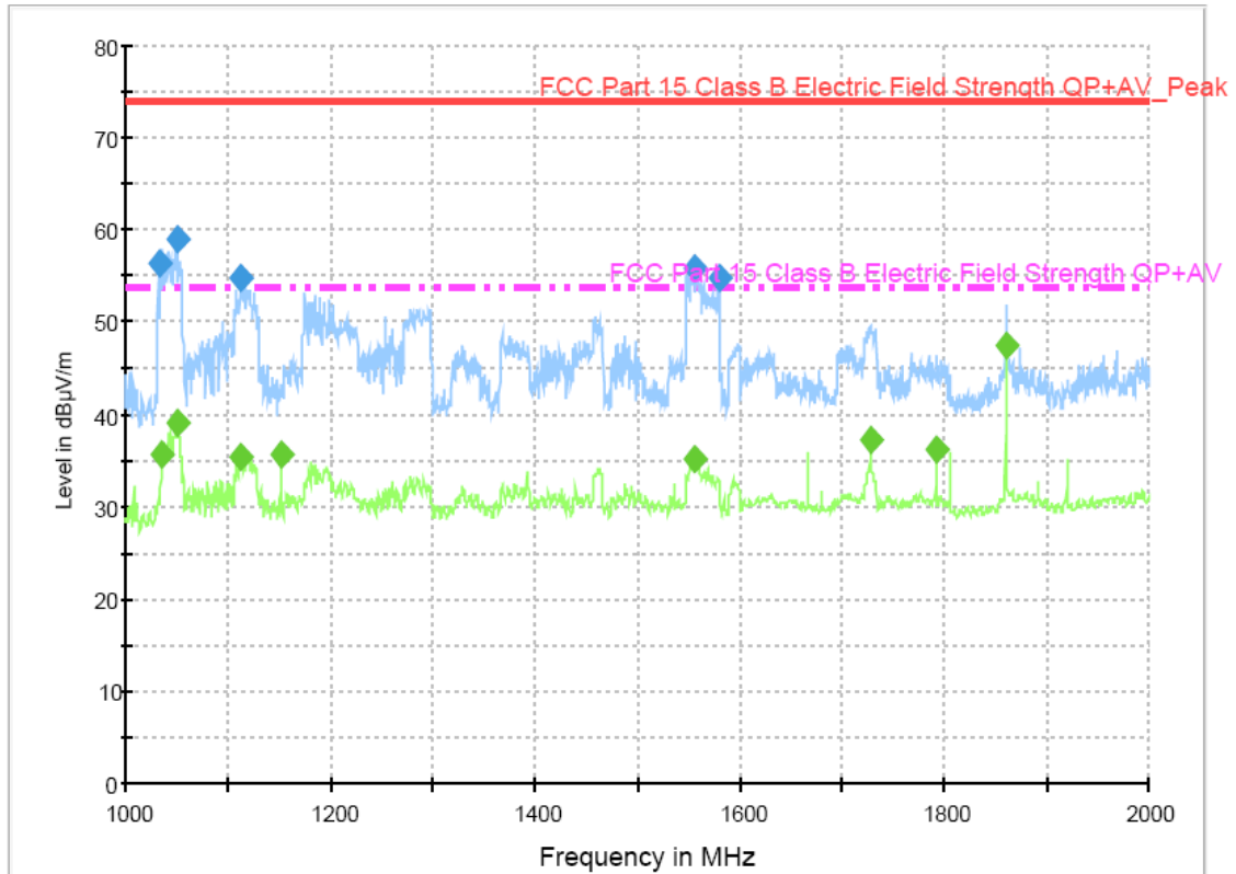
FCC_ESIB_Preamp_RE with Scans
