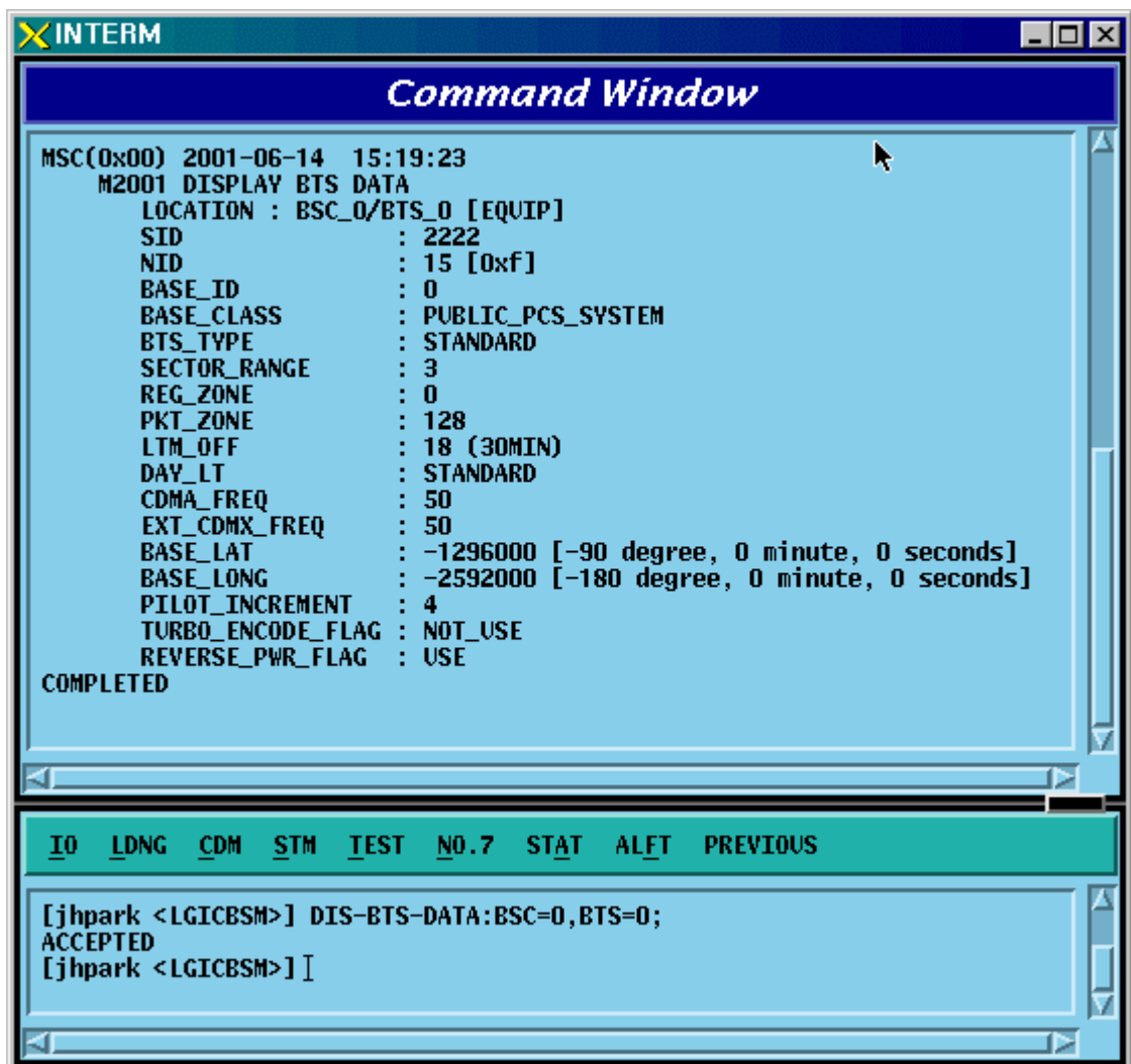
Fig. 4.3-1 BTS Parameter Display
