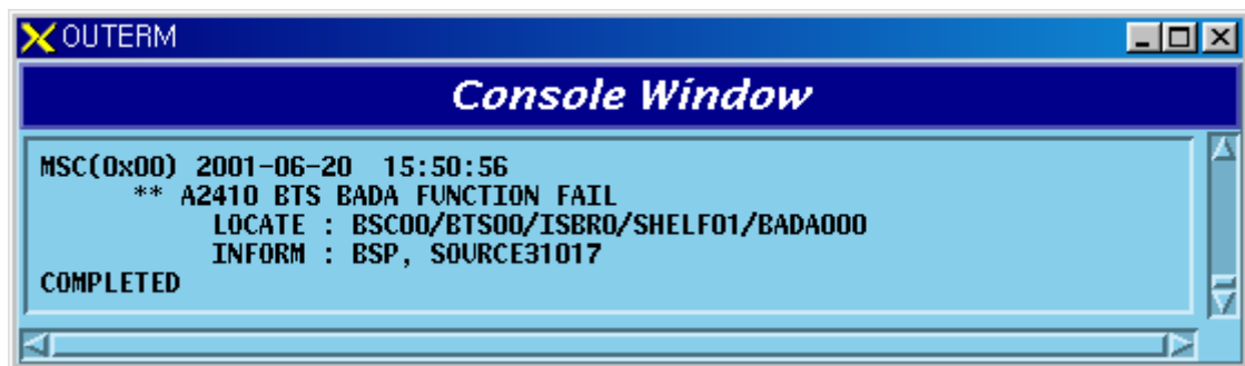
Fig. 5.1-188 BSTB BADA Function Fail
