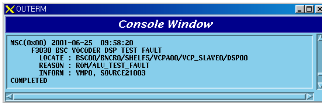
Fig. 5.1-309 Vocoder DSP ROM/ALU TEST Fault
