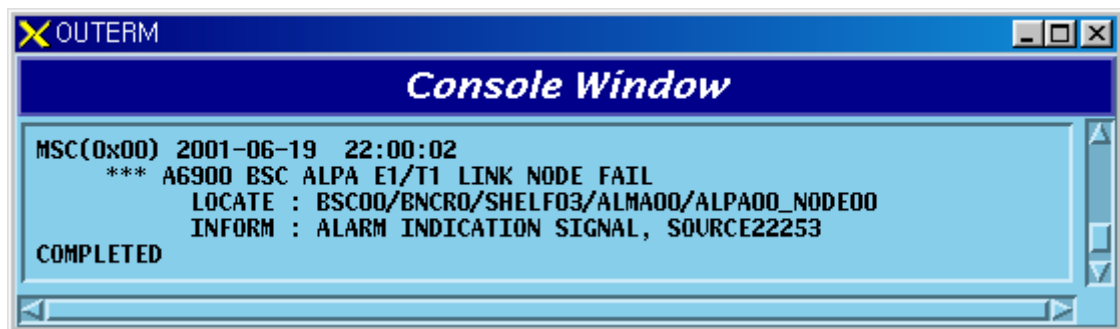
Fig. 5.1-139 ASLB ALPA Link Fail((AIS)
