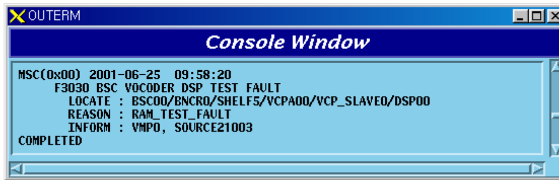
Fig. 5.1-306 Vocoder DSP RAM TEST Fault
