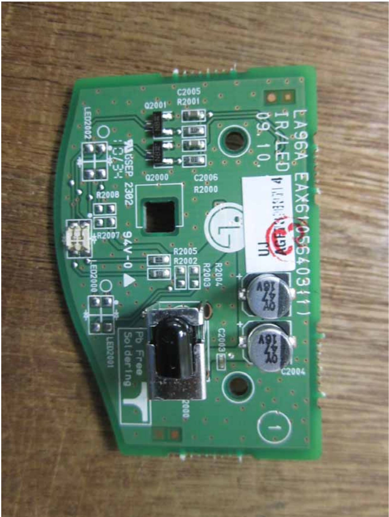
&lt; IR Board Front &gt;
