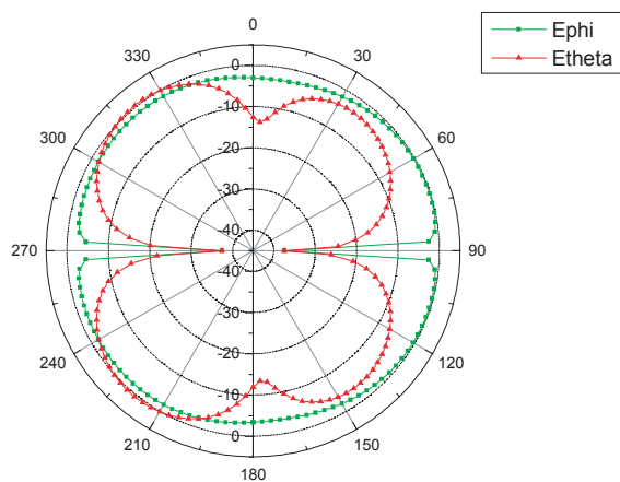
y - z cut (dBi)
