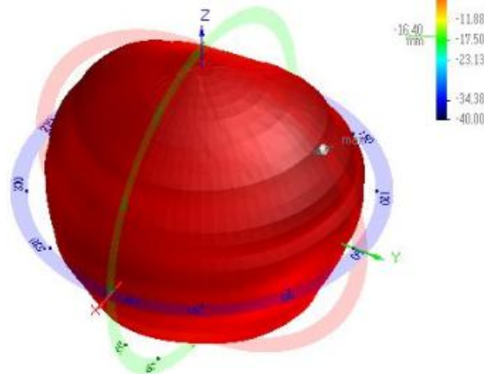
[2442MHz 방사패턴 = EVB 에서 측정]
