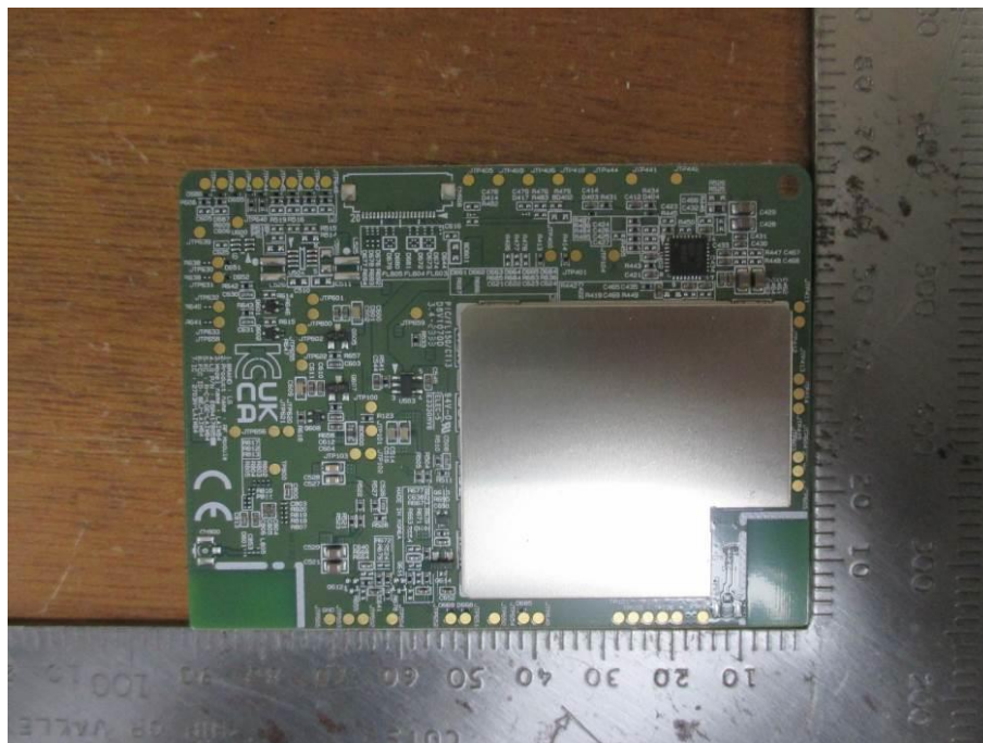
<PCB – Top of Wi-Fi/BT Combo Module >
