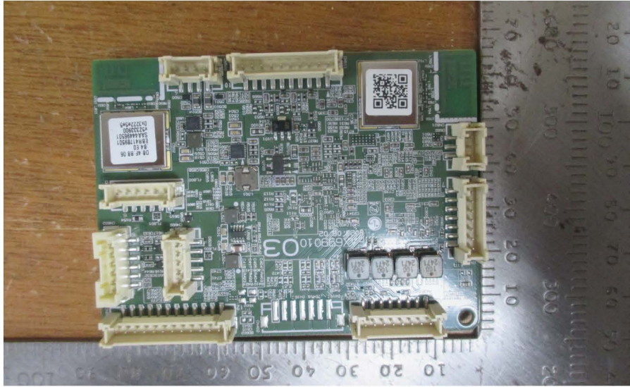
<PCB – Bottom of Wi-Fi/BT Combo Module >
